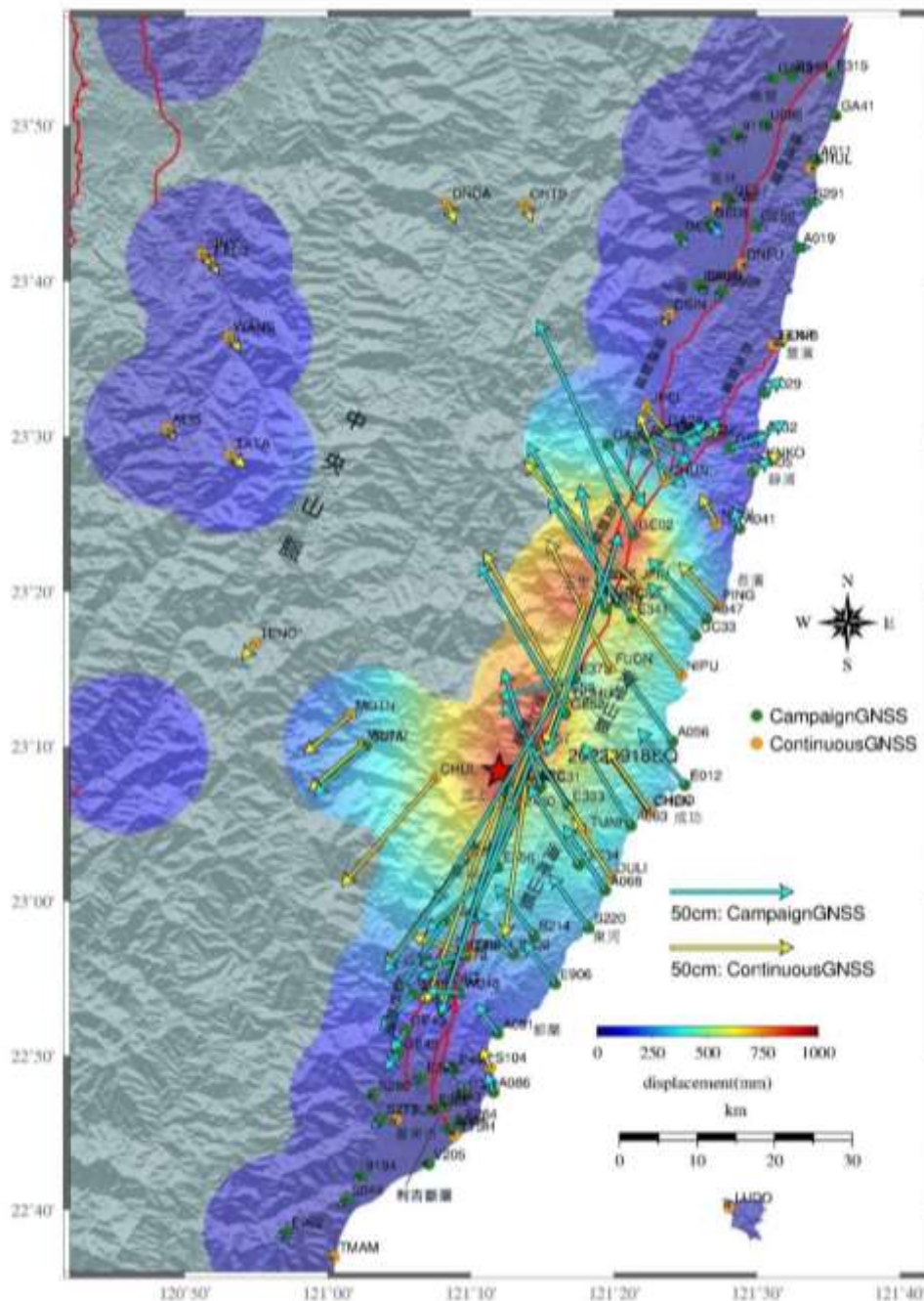
圖 11、0918 池上地震之 GNSS 測量水平方向同震位移分布圖，箭頭代表水
