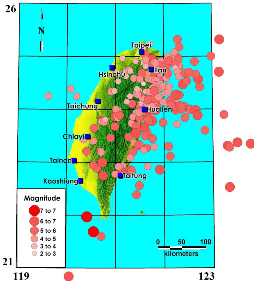
圖 3 DANB 井下站在 2005 年 10 月至 2013 年 10 月所收錄臺灣地區地震之震央分佈。
