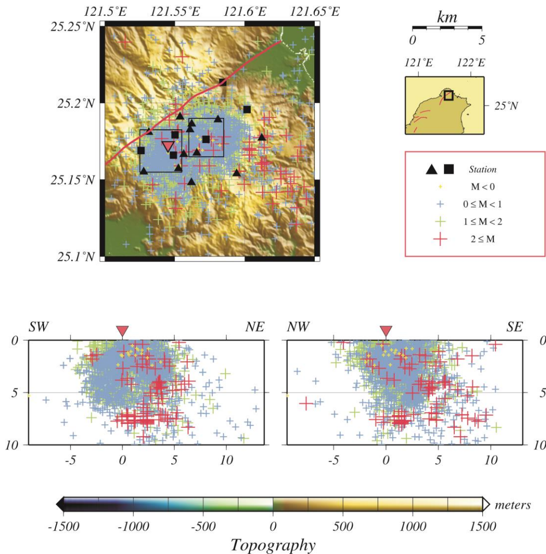
圖5 大屯山地區過去數年中之微震活動分布。資料起自2003年5月至2013年6月於左上圖中的兩個黑框分別表示七星山(西邊)與大油坑(東邊)地區。
