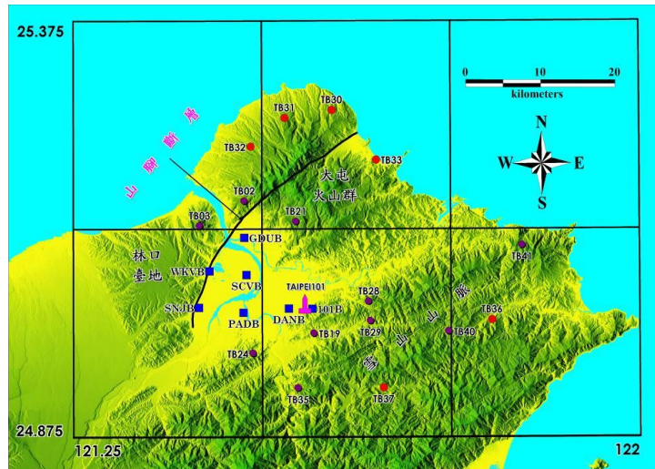
圖 1 大台北地區寬頻地震觀測網的測站位置分佈，紅色實心圓是 6 個地表固定站，藍色方塊是 7 個井下站（含 101B，地球所建立），深棕色實心圓是 10 個臨時站（地球所建立）。
