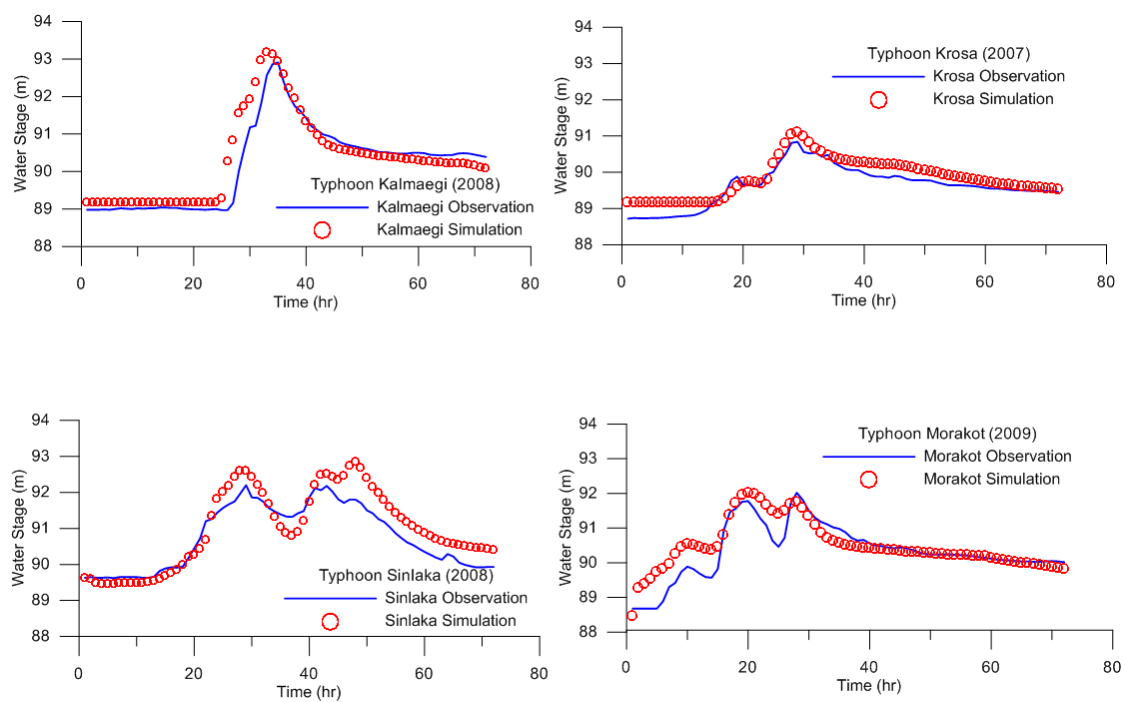
圖 2 歷史颱風事件之烏溪流域烏溪橋水位模擬比較圖
