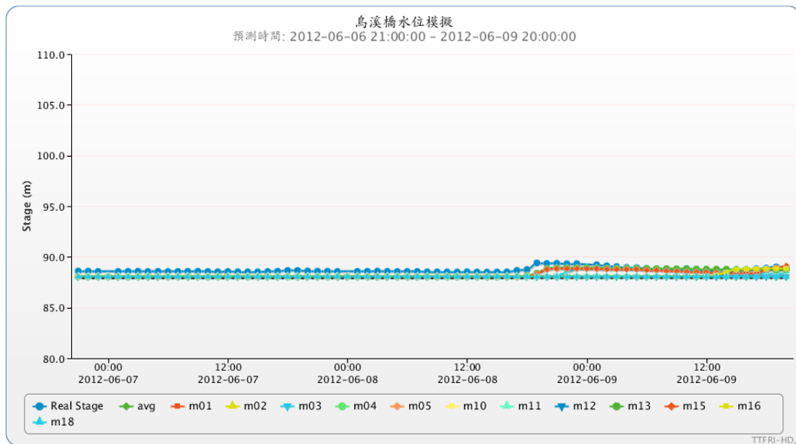
圖 4 烏溪橋即時水位模擬與觀測結果
