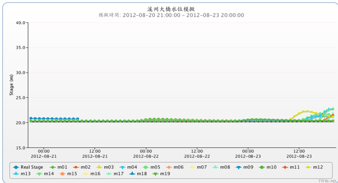
圖 5 溪州大橋即時水位模擬與觀測結果
