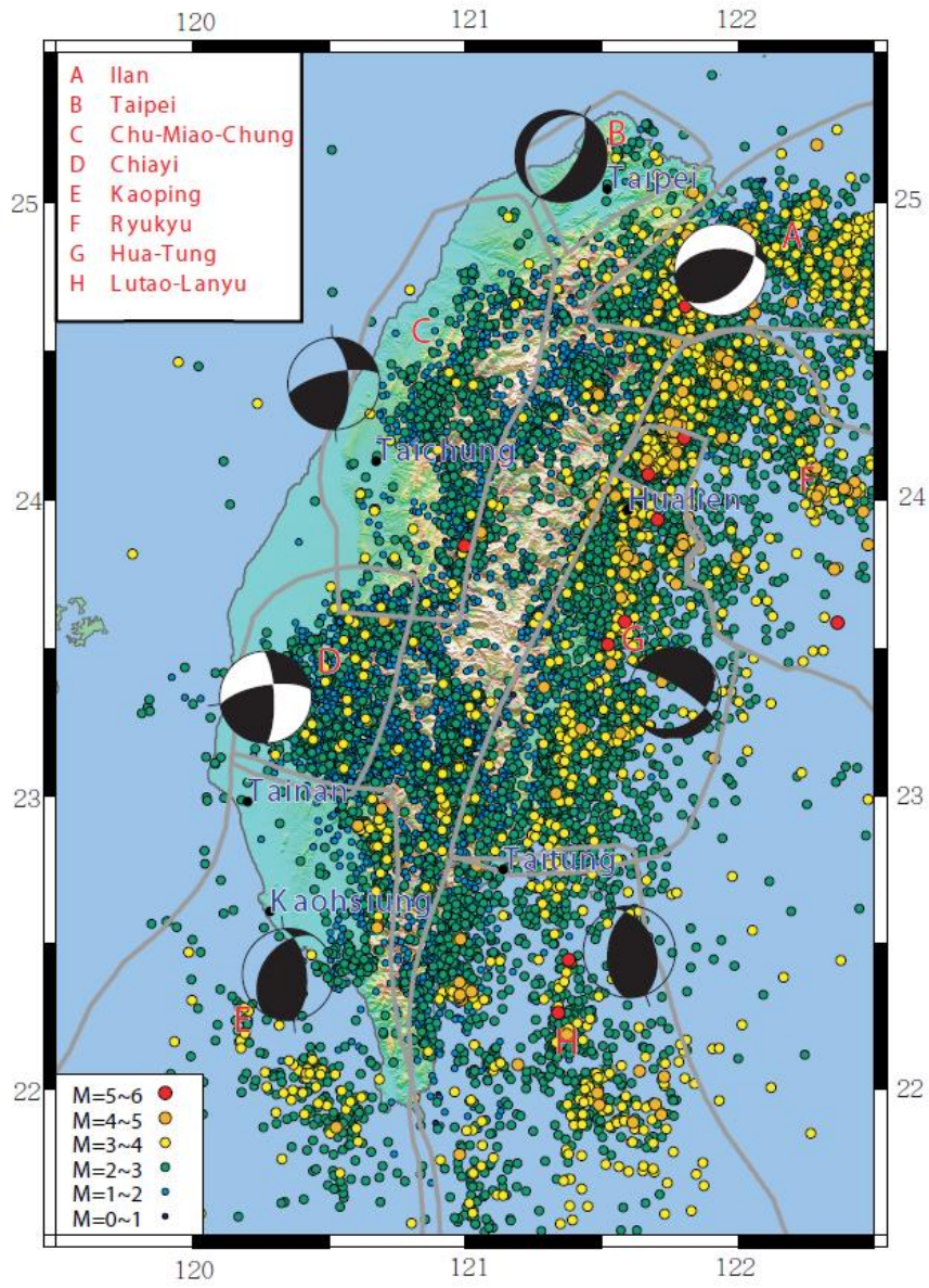
圖 4-1: 2010/07-2011/06 各構造分區的大地應力方向。
