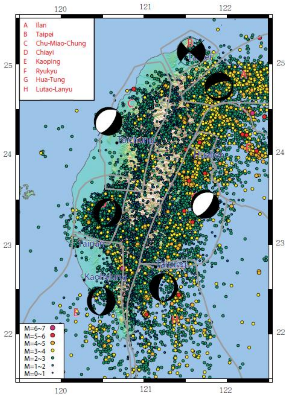
圖 4-2: 2011/0-2011/12 各構造分區的大地應力方向。
