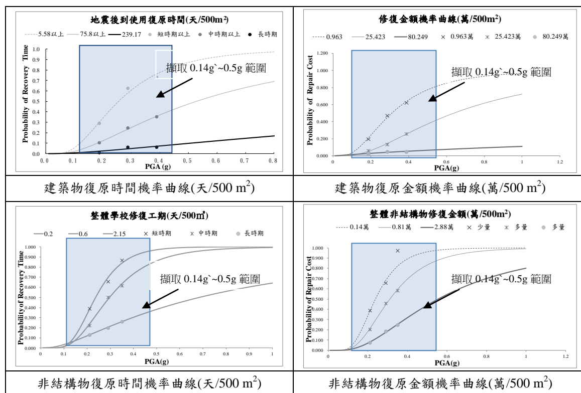
圖 1 復原時間及復原金額機率曲線圖
