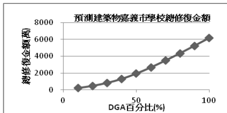
圖 6 預測建築物嘉義市學校總修復金額圖
