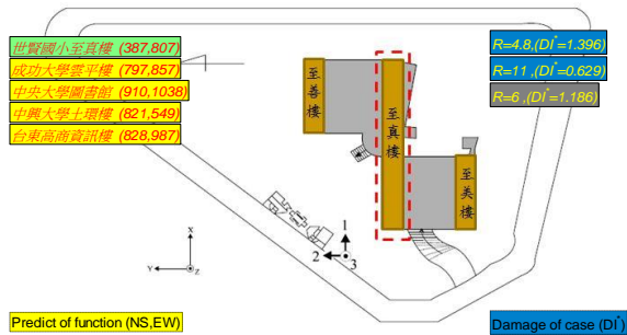
圖 10 世賢國小至真樓於 475 年回歸期人工地震之最大加速度預估與震損預估圖
