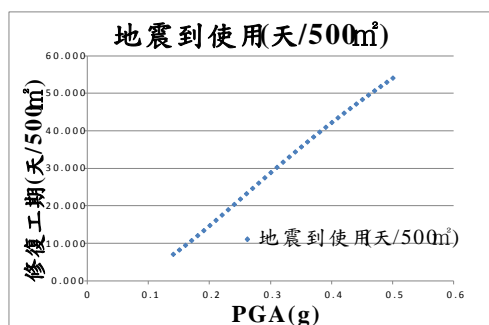
圖 4 建築物復原時間圖
