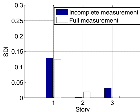
圖 18 不足量測與全量測之損壞評估結果比較
