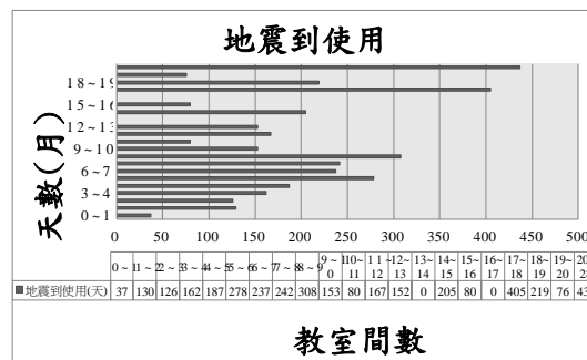
圖 5 嘉義市學校建築物之工期分佈圖
