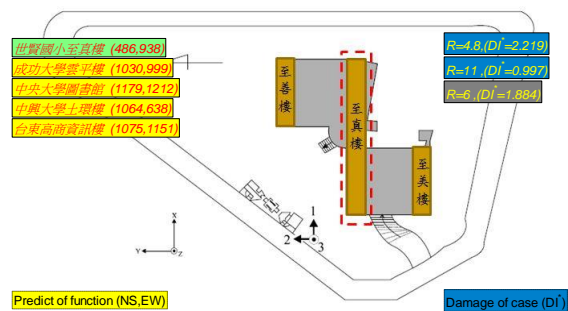
圖 13 世賢國小至真樓於 2500 年回歸期人工地震之最大加速度預估與震損預估圖
