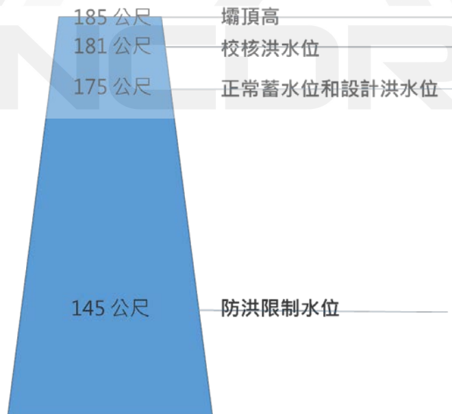
圖 49、長江三峽大壩水位高度說明（災防科技中心繪製）[5]
