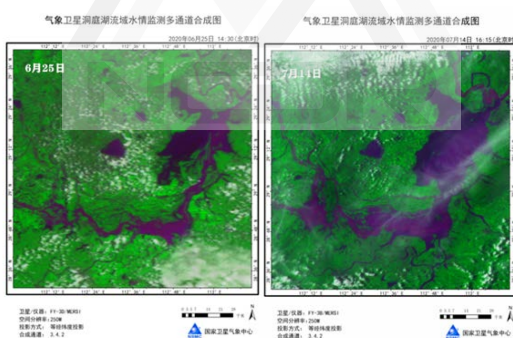
圖 12、洞庭湖 6 月 25 日與 7 月 14 日衛星監測影像，圖中深藍色為水體 (資料來源：中國國家衛星氣象中心) [6]
