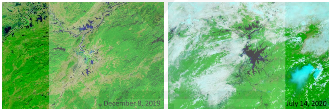
圖 9、鄱陽湖災前（2019 年；左圖）災中（2020 年；右圖）衛星影像 圖中深藍色為水體。（資料來源：National Aeronautics and Space Administration (NASA)) [9]
