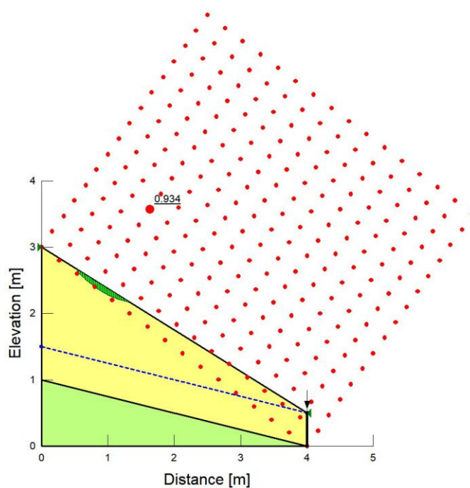
圖 5.1-6 邊坡覆蓋至擋土構造後方時，地下水位上升 50cm 模擬剖面圖
