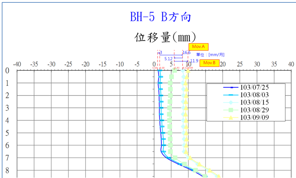
圖 2.3-13 103/07/25~103/09/09 BH-5 孔口變位與變位速率(水保局 2014)
