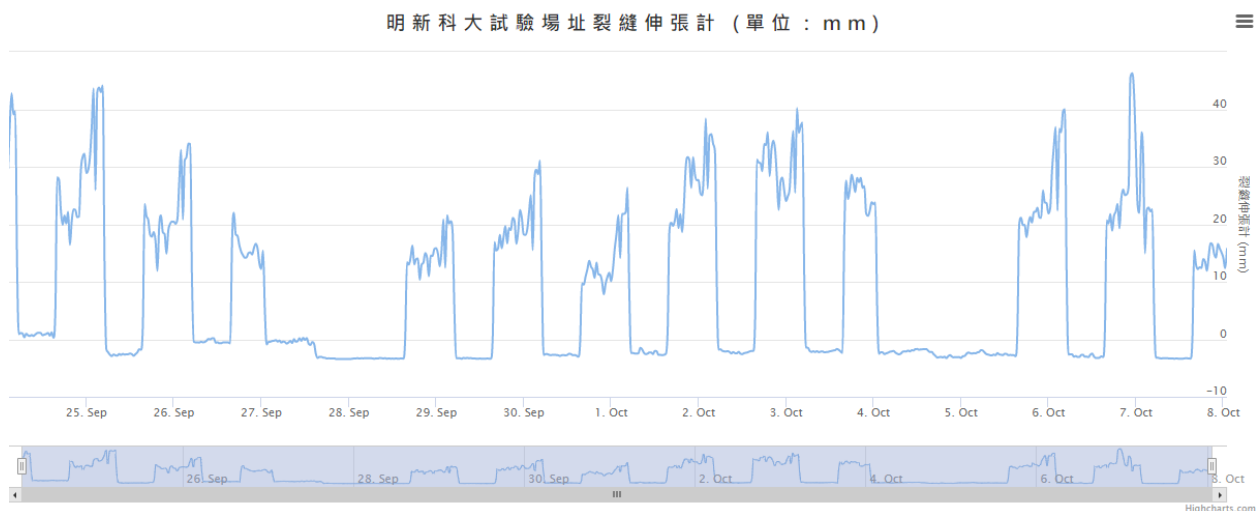
圖 6.2-5 裂縫伸張計的監測資料
