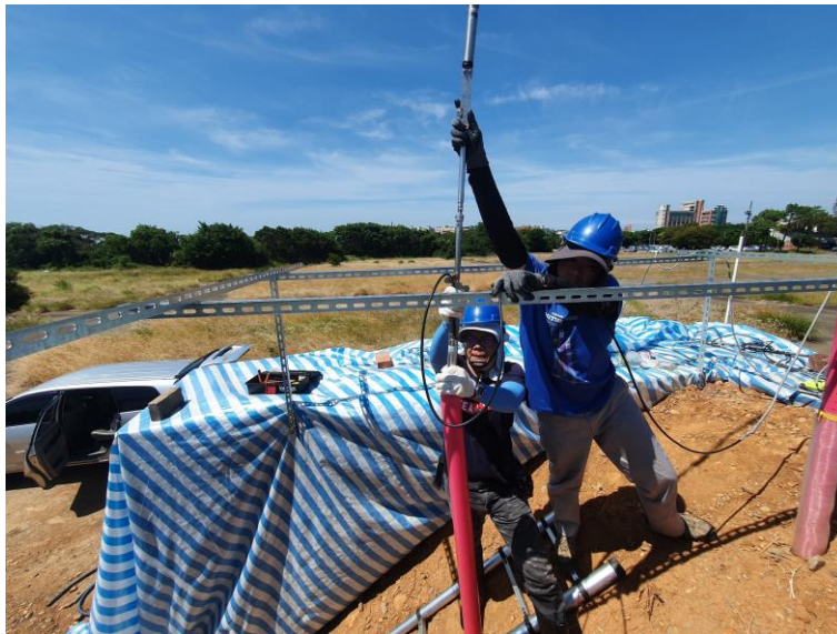
圖 3.2-9 定置型地中傾斜儀於模擬邊坡裝設
