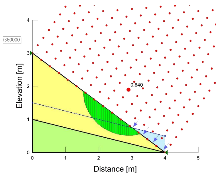
圖 5.1-5 邊坡下水位上升 50cm 且於擋土構造後方蓄積模擬剖面圖
