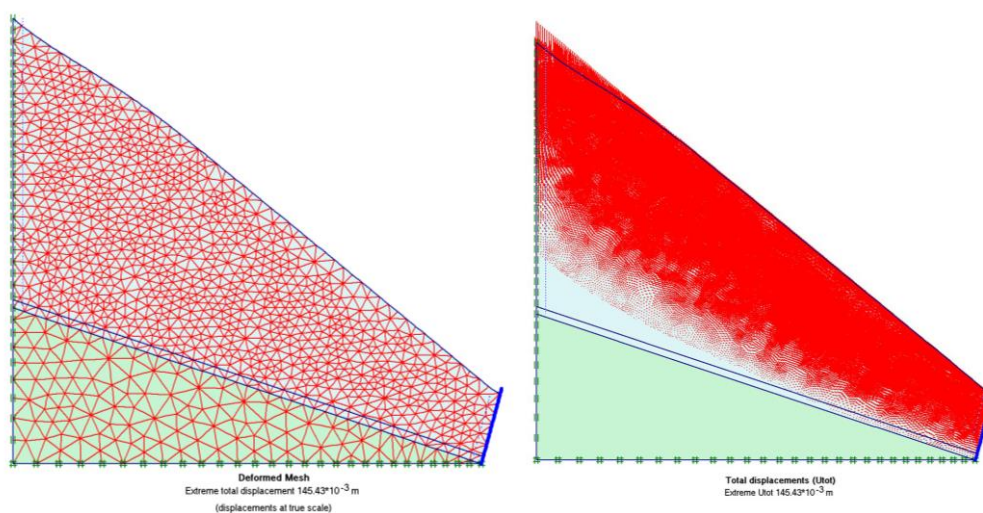
圖 5.2-2 有限元素法之水平變位分佈圖
