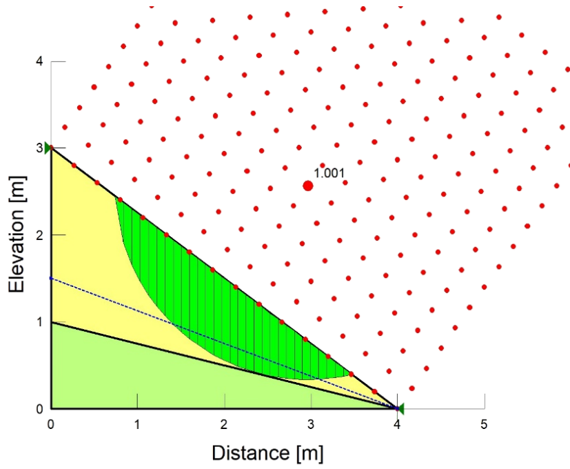
圖 5.1-3 邊坡下水位上升 50cm 模擬剖面圖
