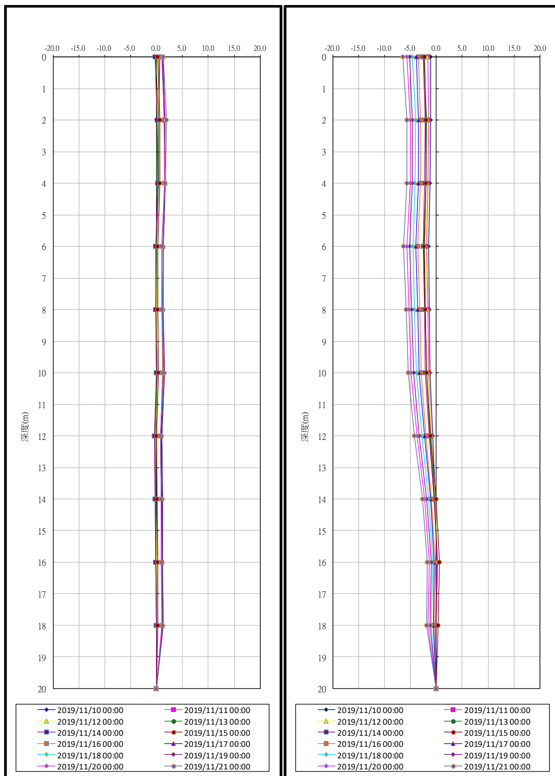
圖 2.2-6 自動量測傾度管紀錄
