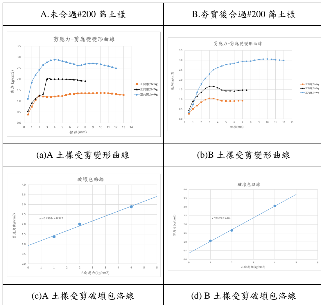
圖 5.1-1 重模土樣力學試驗成果
