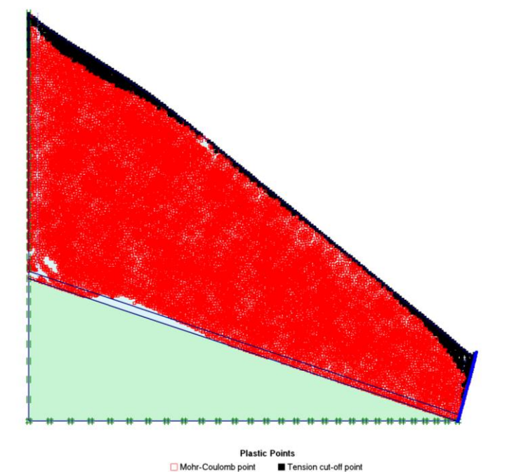
圖 5.2-3 有限元素法破壞點分佈圖
