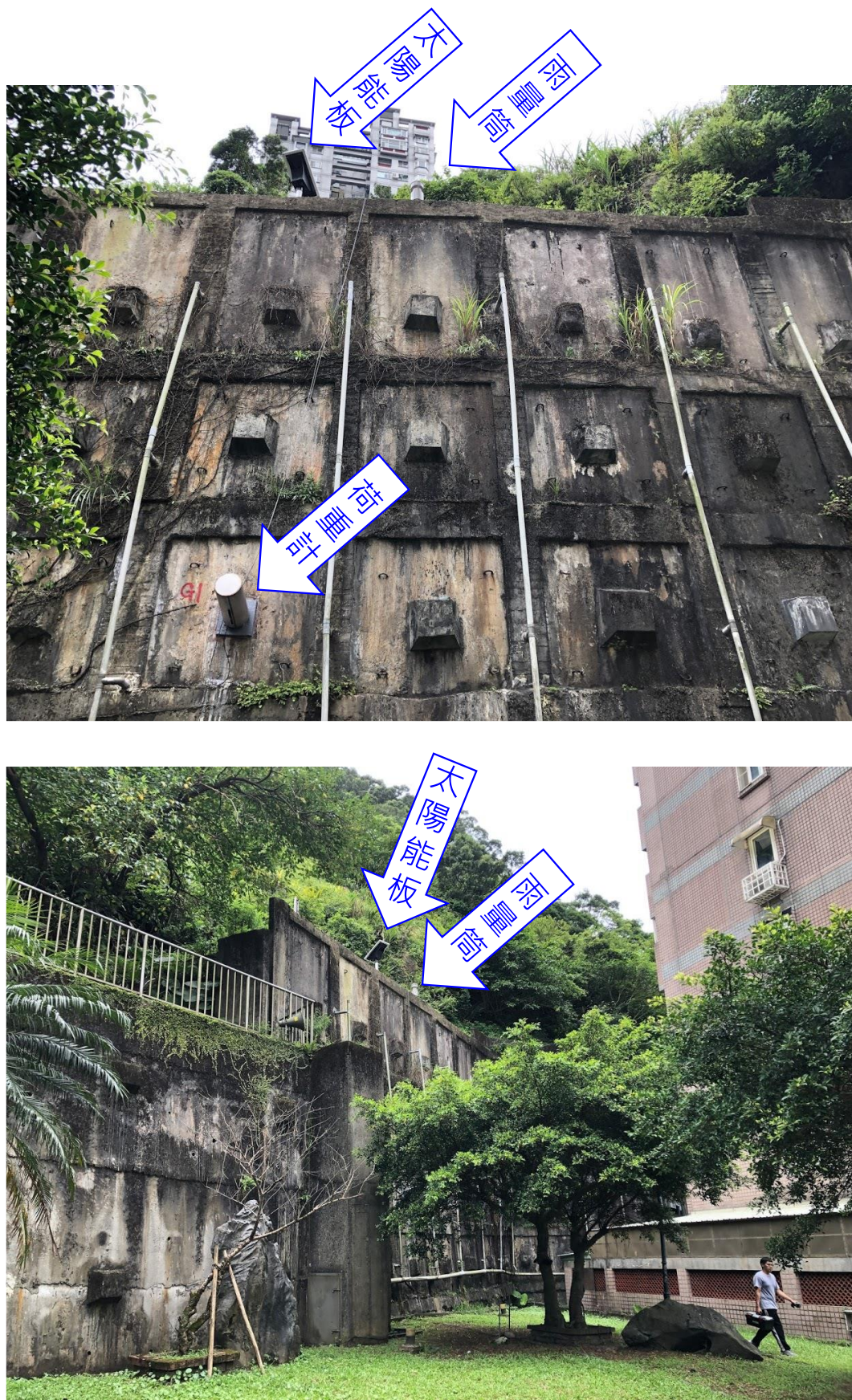
圖 2.2-1 現場監測設備裝設完畢後照片
