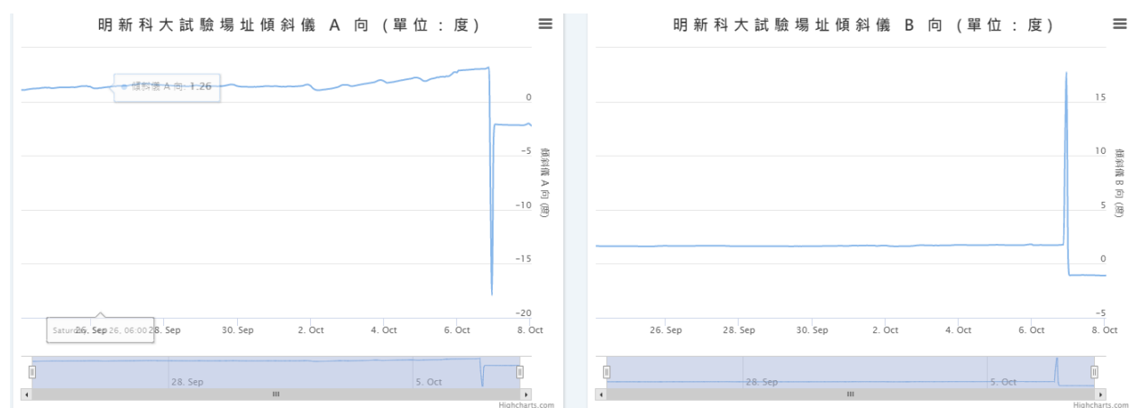
圖 6.2-9、土坡下傾斜儀監測數據
