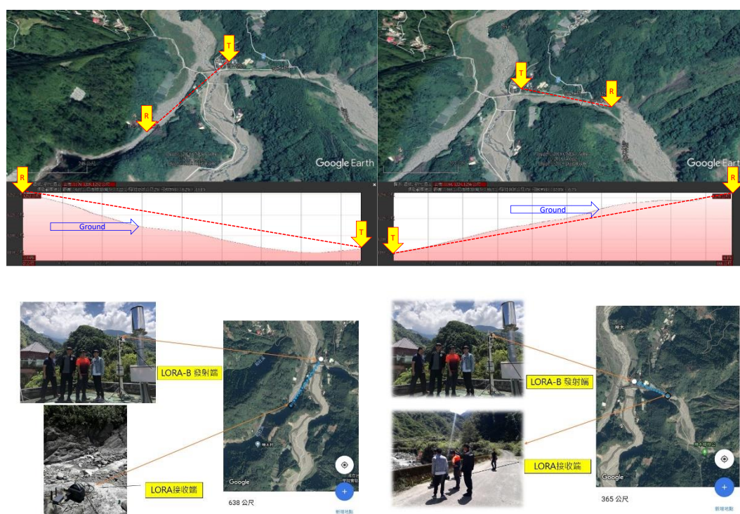
圖 2.3-2 於南投縣信義鄉神木村土石流觀測站進行 LoRa 傳輸試驗狀況(水保局 2018)
