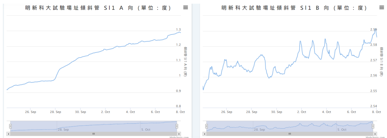
圖 6.2-6 土坡中段傾斜管 S11 監測數據
