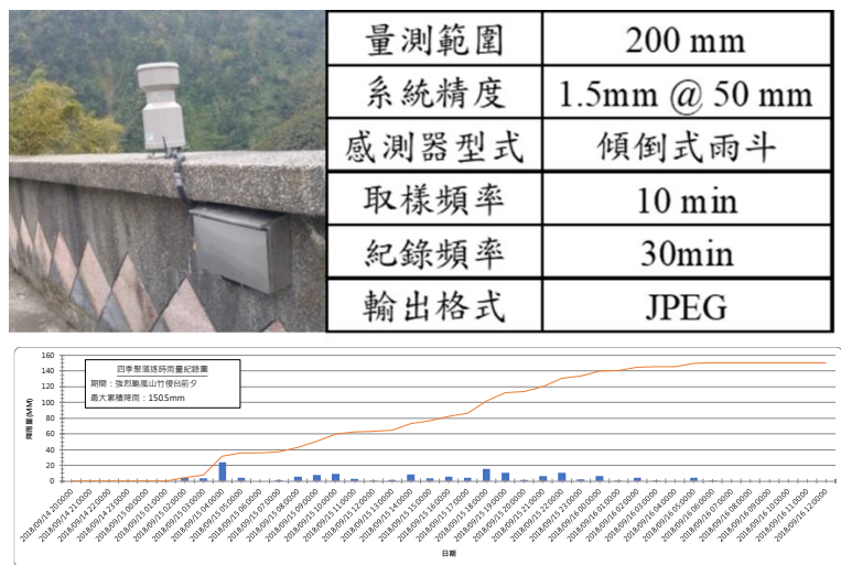
圖 2.2-3 本研究採用之雨量監測系統與成果示意圖
