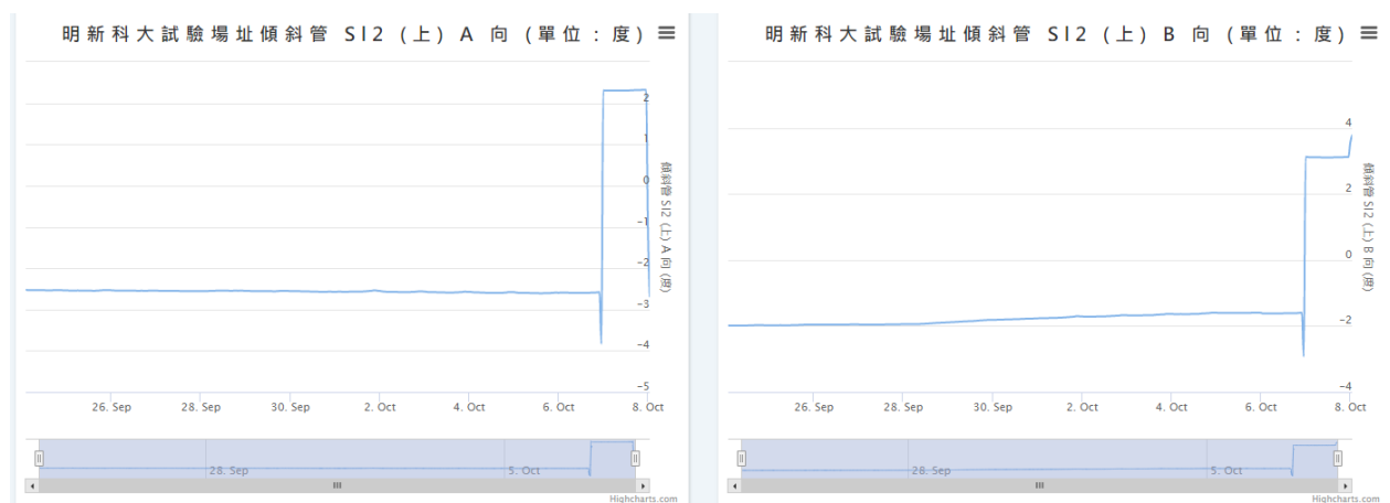
圖 6.2-7、土坡上方傾斜管 S12(上) 監測數據
