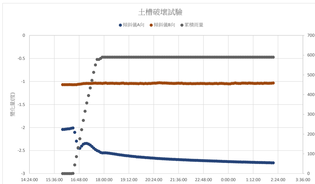
(c) 累積降雨與擋土結構變化關係
