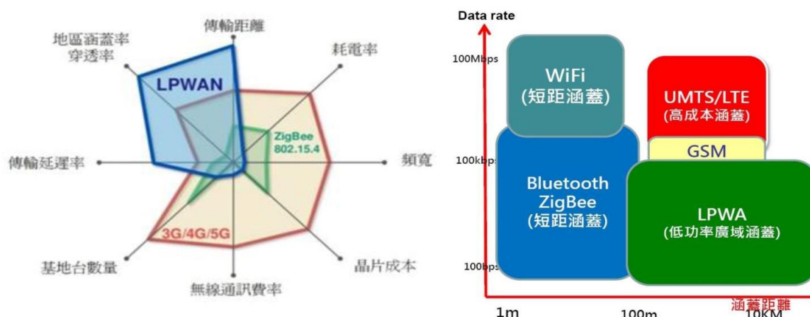
圖 2.3-7 LPWAN 廣域物聯網路之優勢及 IoT 頻譜分析
