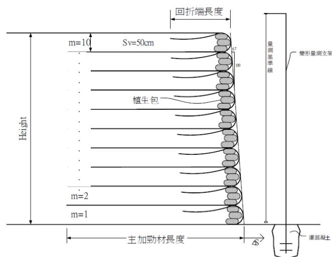
圖 2.4-2 大尺寸加勁擋土牆剖面示意圖(楊錦裕 2004)
