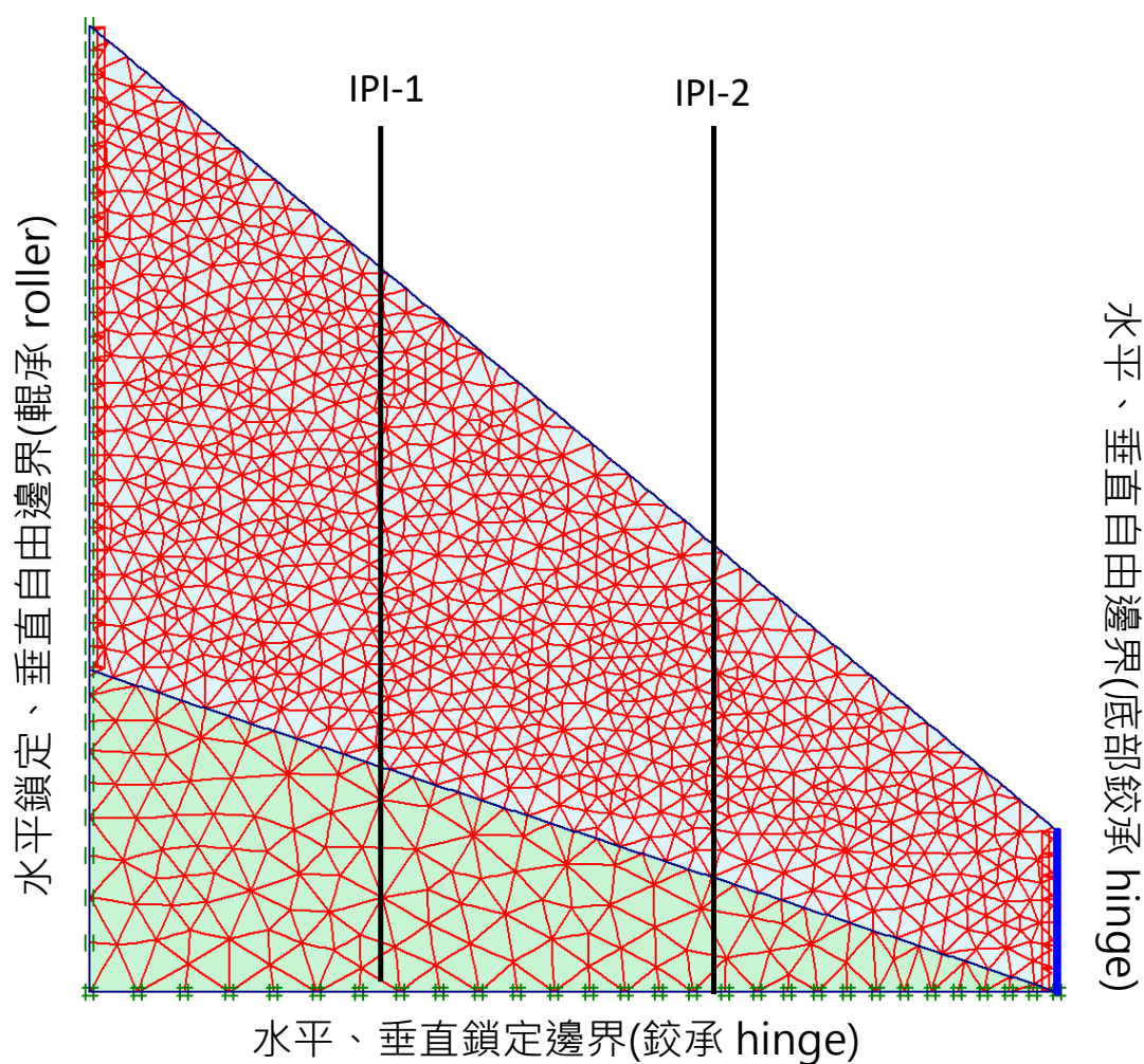
圖 5.2-1 數值模擬模型 AA'剖面圖
