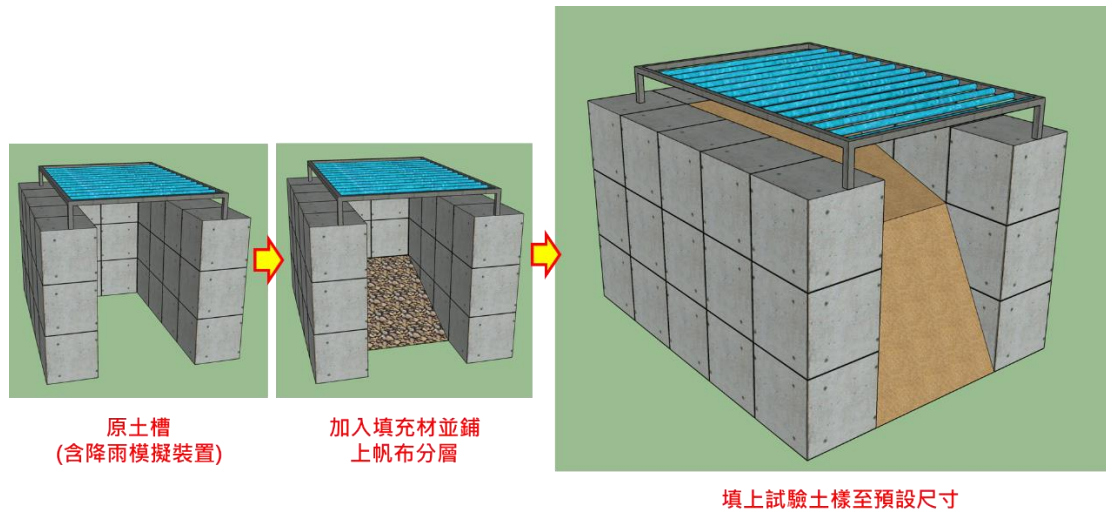
圖 3.1-2 土槽配置示意圖
