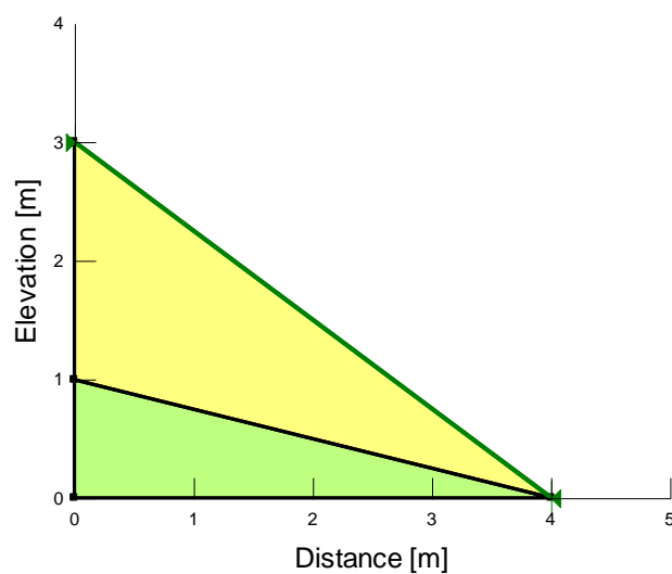
圖 5.1-2 邊坡穩定模擬剖面圖
