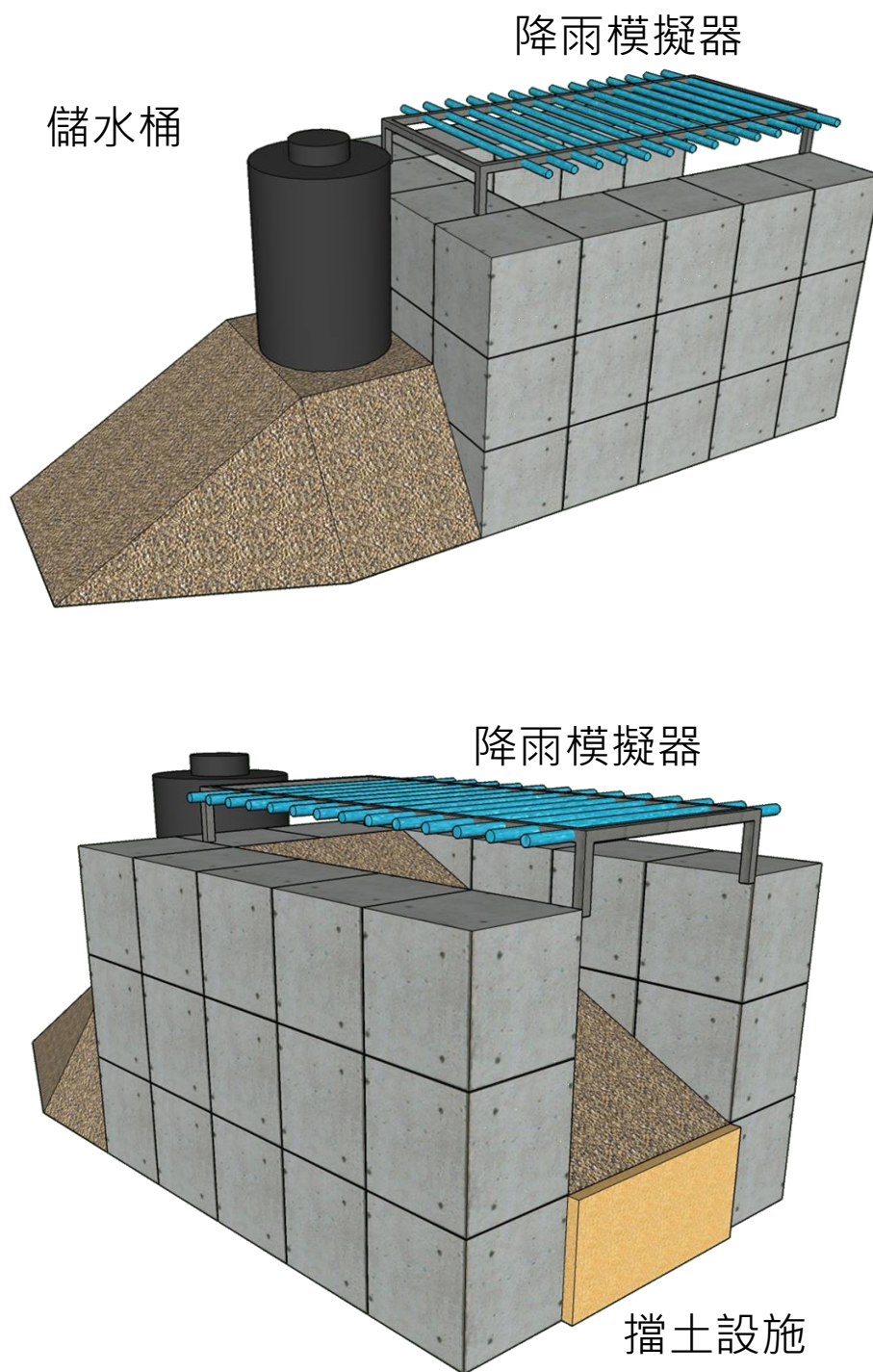
圖 5-1 大尺寸邊坡模型示意圖
