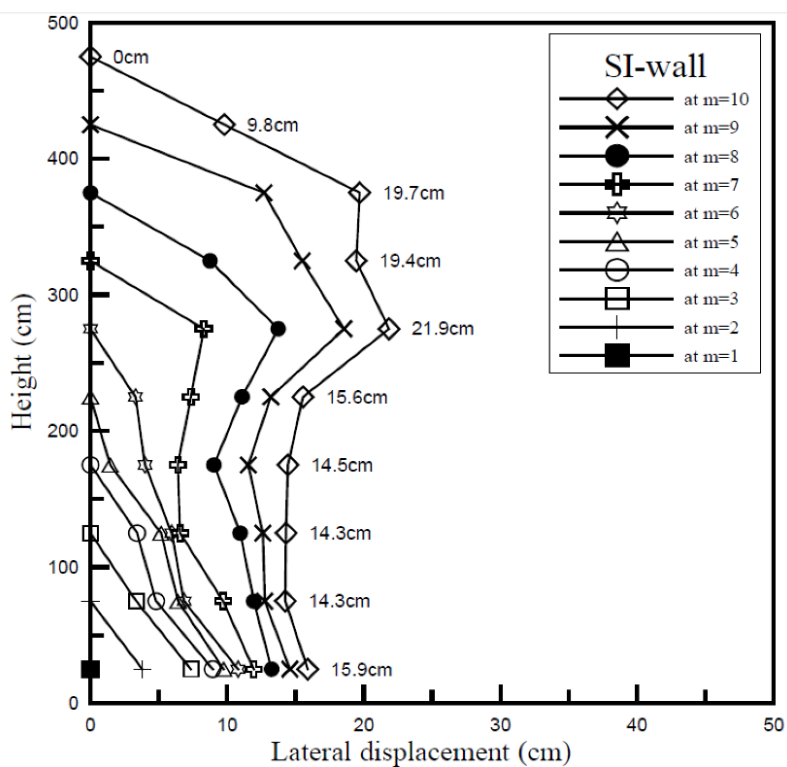
圖 2.4-4 大尺寸加勁擋土牆構築過程即已開始變形(楊錦裕 2004)
