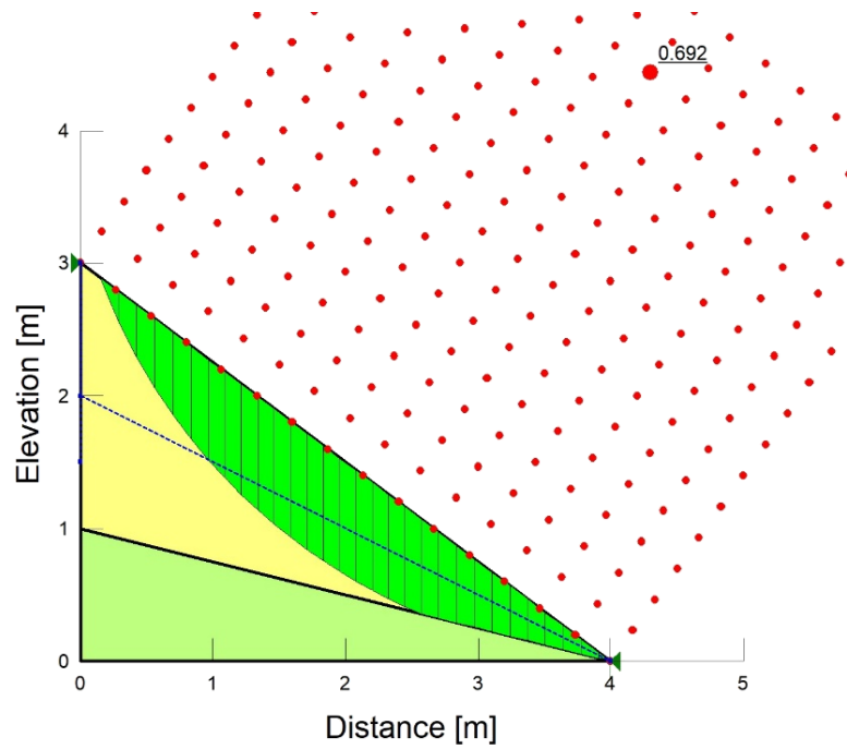
圖 5.1-4 邊坡下水位上升 100cm 模擬剖面圖
