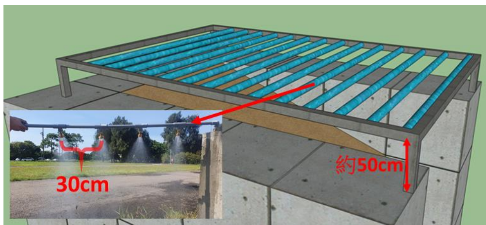
圖 4.2-2 降雨模擬裝置示意圖
