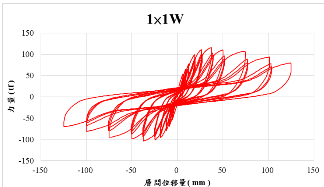
圖 4.1 1x1W 試體遲滯迴圈
