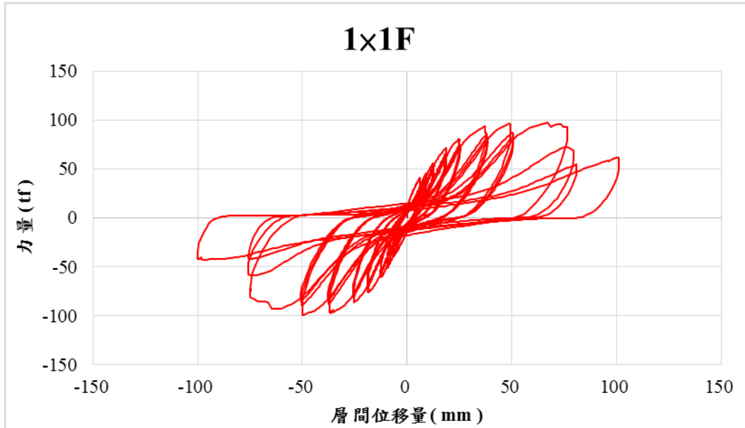
圖 4.5 1x1F 試體遲滯迴圈
