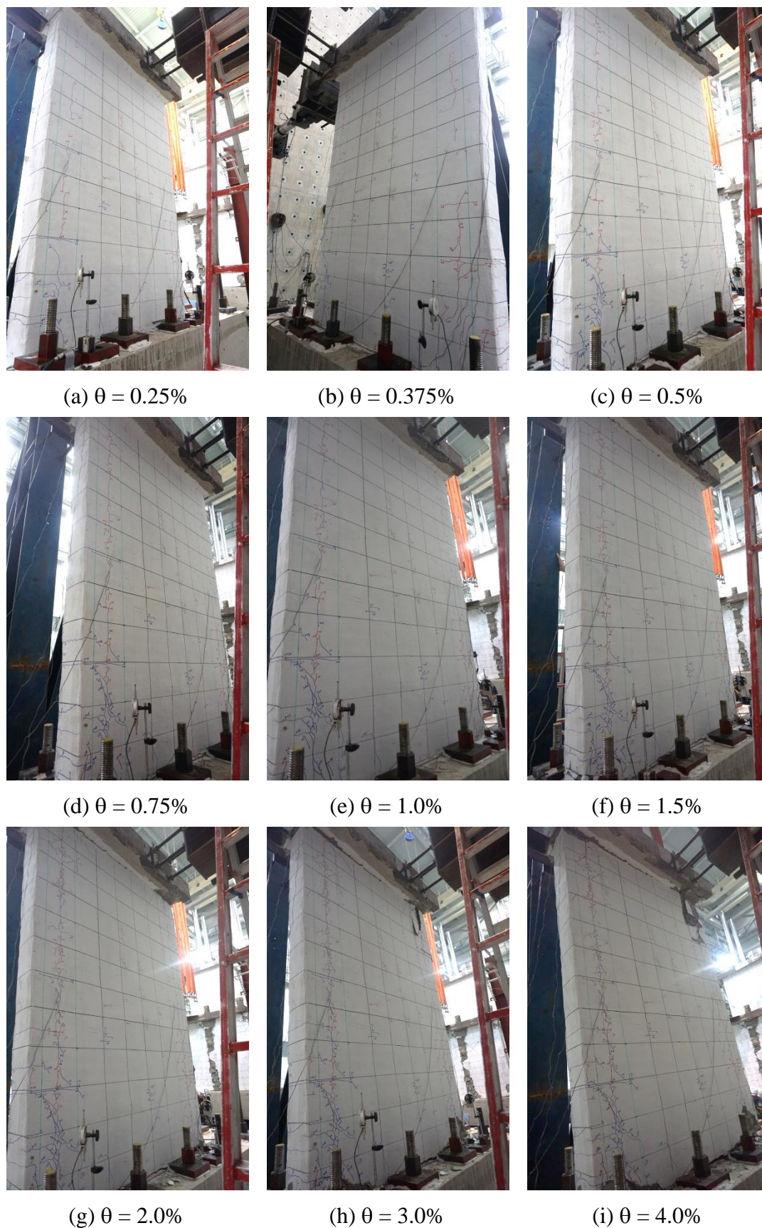
圖 4.7 1x1F 試體不同層間位移角試體破壞情況
