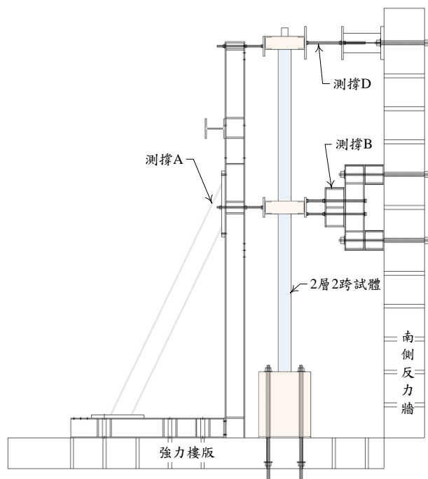
(c) 側視圖
