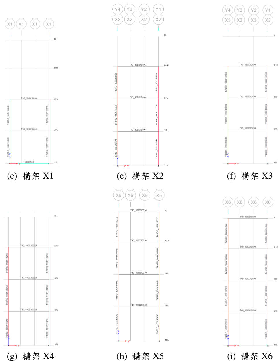
圖 5.9 分析模型構架立面圖(續)
