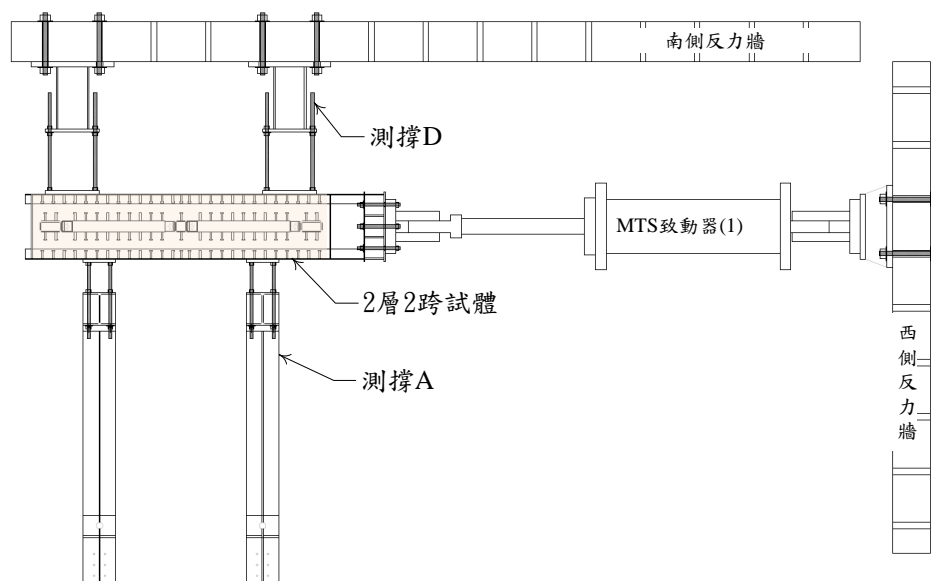
(b) 上視圖
