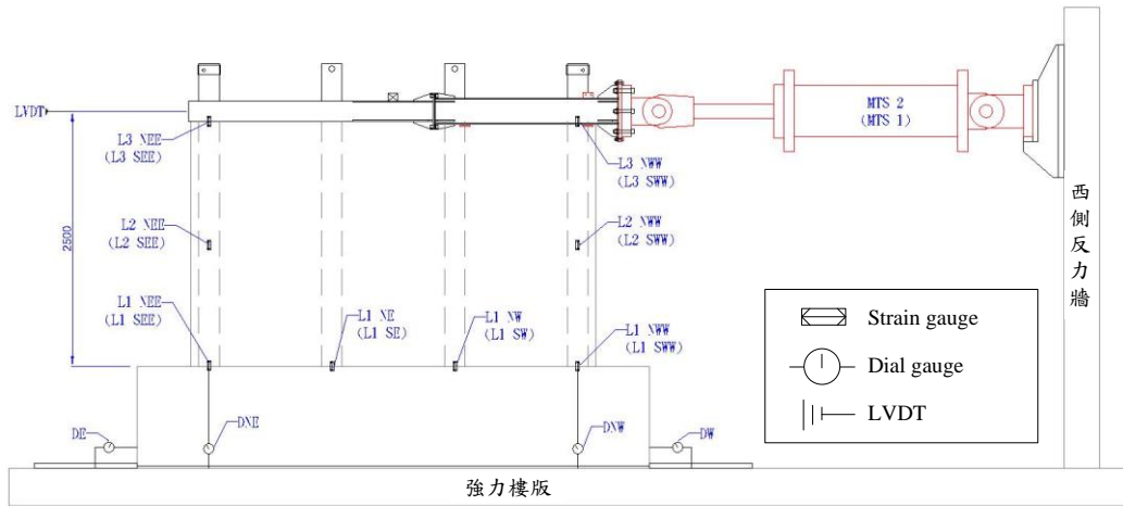
圖 3.20 1x3 試體測計配置
