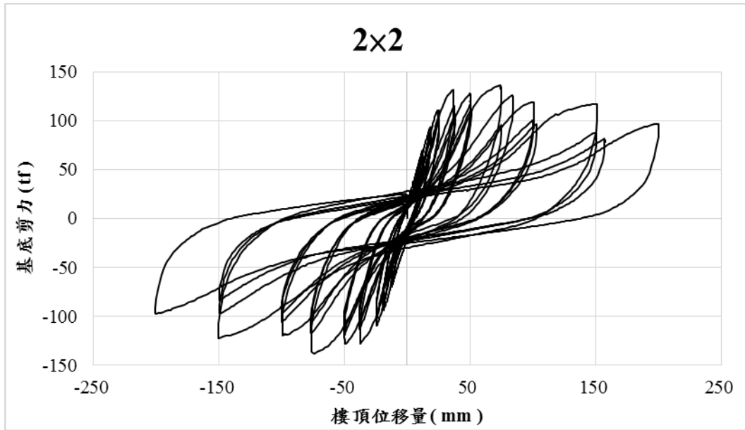
圖 4.19 2x2 試體遲滯迴圈
