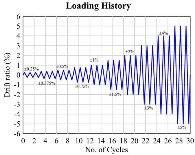
圖 3.18 加載歷程圖 (資料來源：本研究製作)
