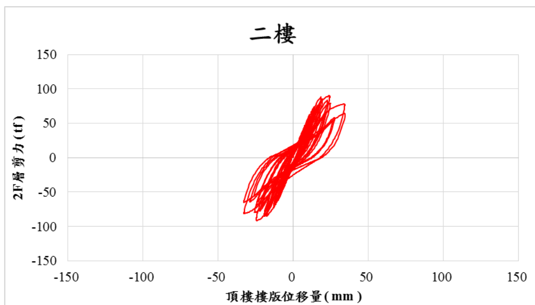
(a) 二樓
