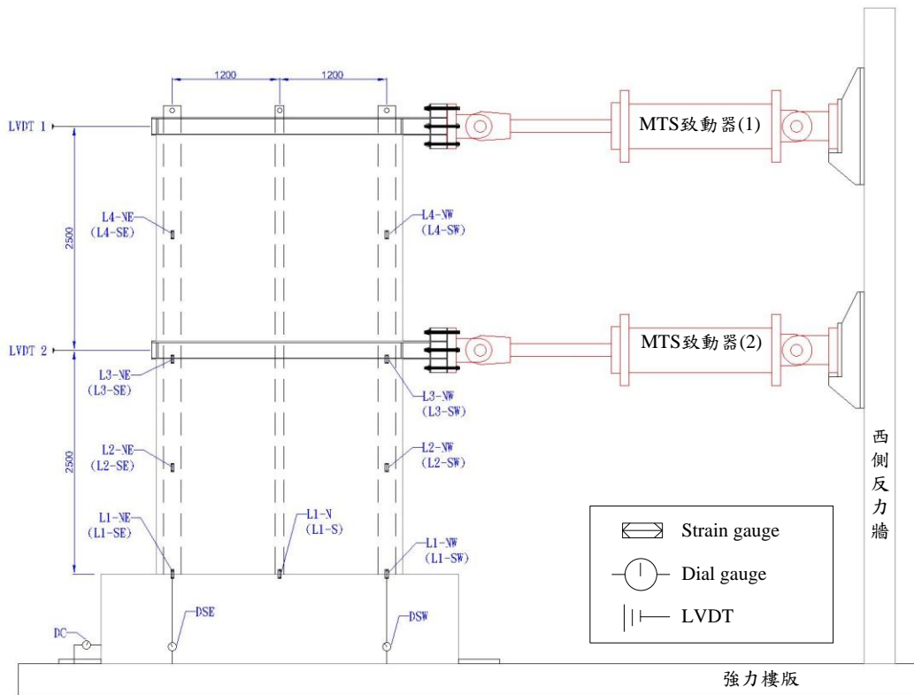
圖 3.21 2x2 試體測計配置
