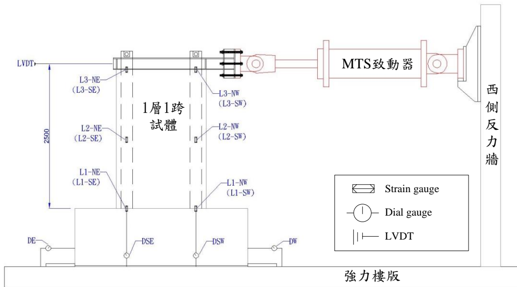
圖 3.19 一層一跨試體測計配置 (資料來源：本研究製作)
