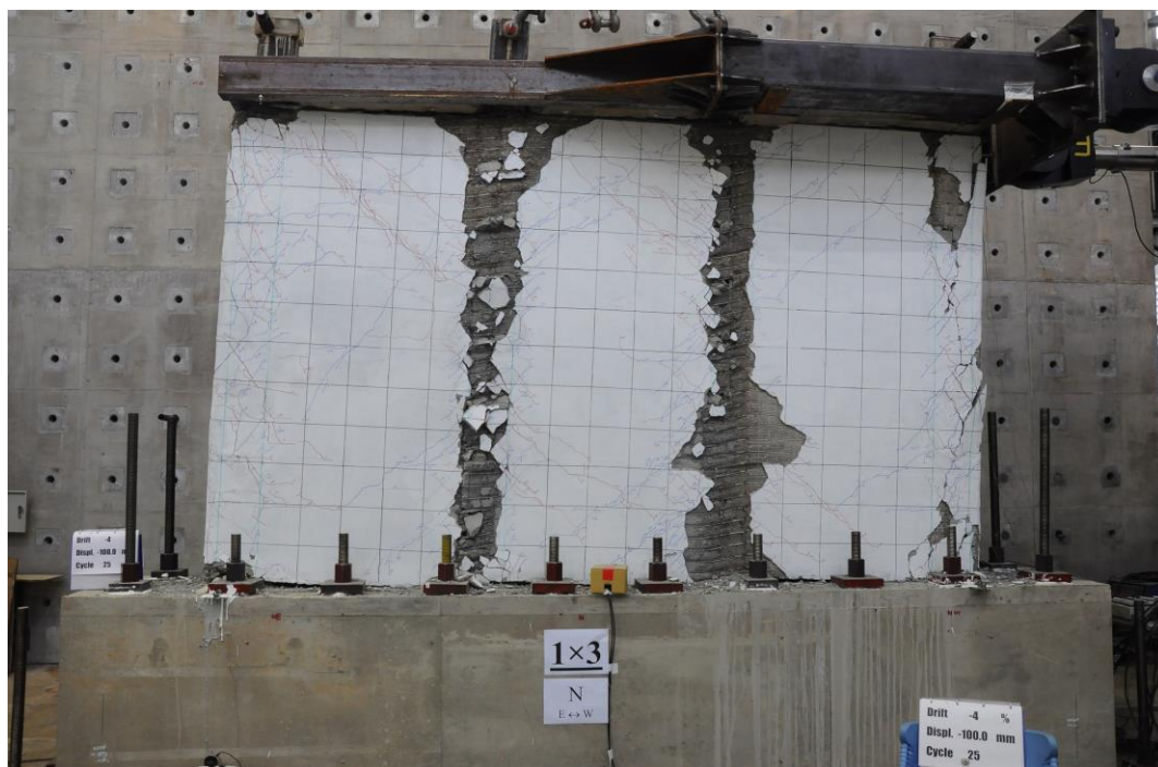
圖 4.15 1x3 試體不同層間位移角試體破壞情況(續)
