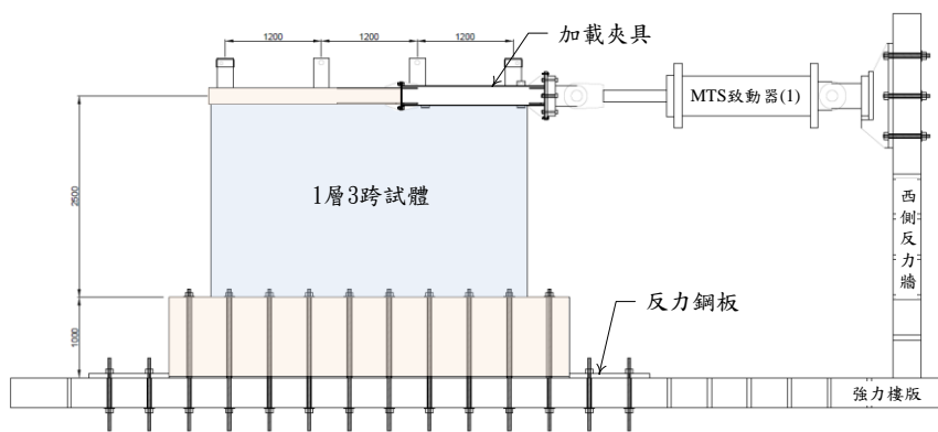
(a) 正視圖
