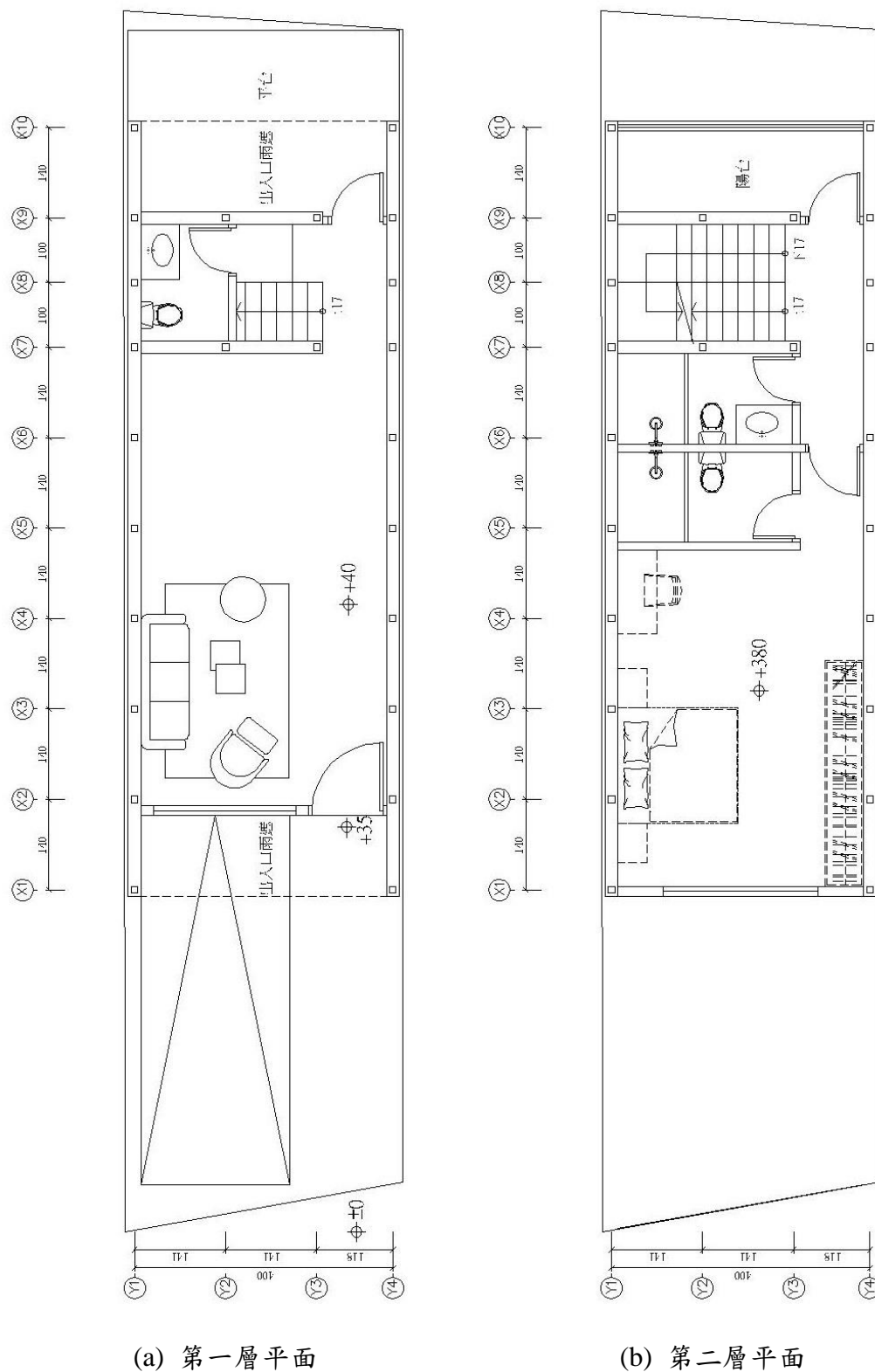
圖 5.4 案例建築圖
