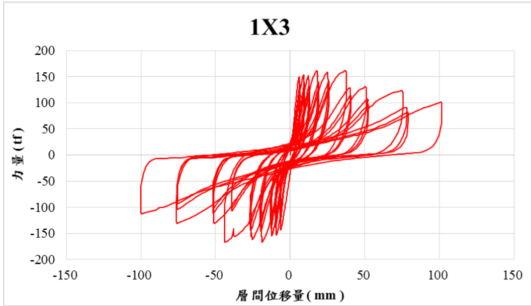
圖 4.13 1x3 試體遲滯迴圈
