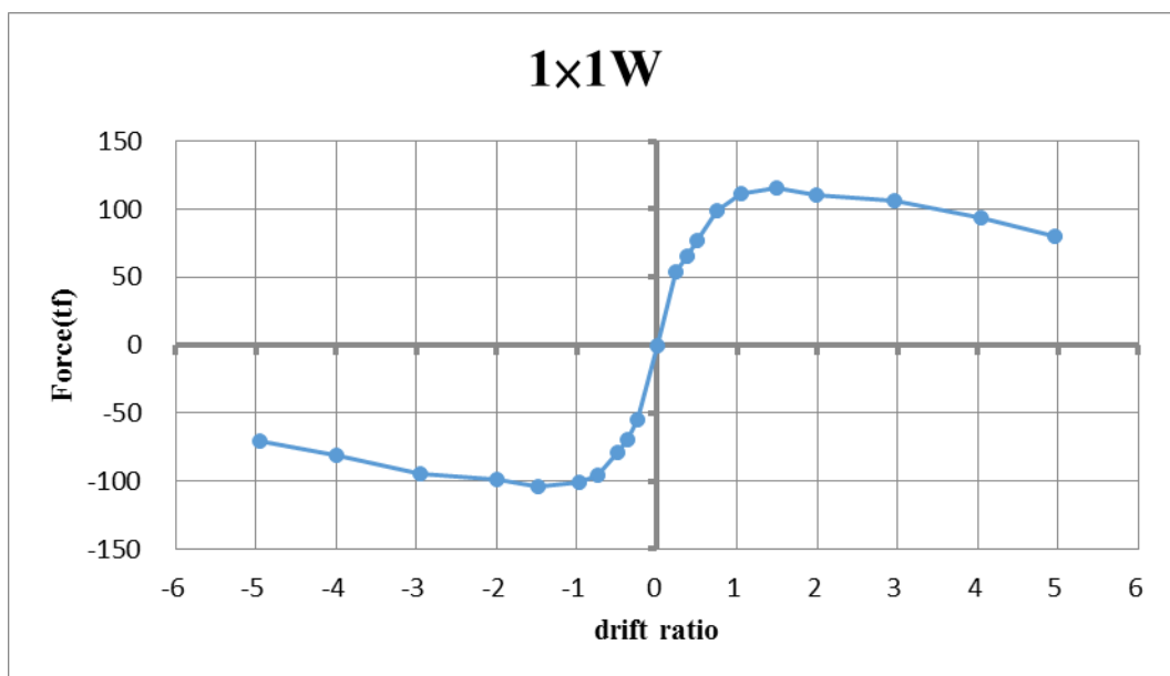
圖 4.2 1x1W 試體遲滯迴圈包絡線
