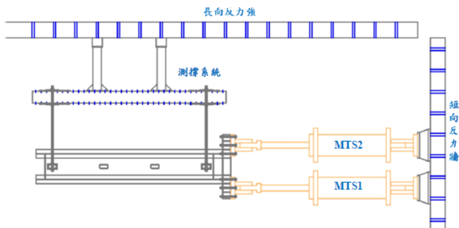
上視圖
