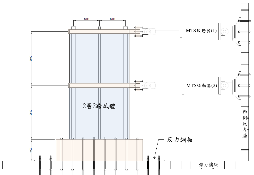
(a) 正視圖
