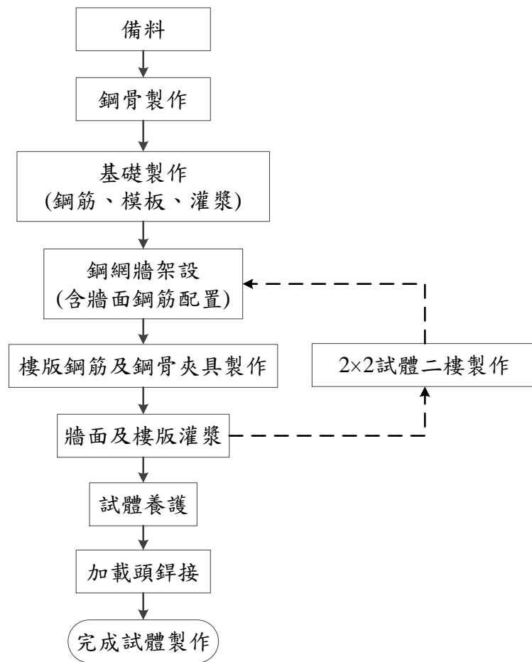
圖 3.10 試體製作流程
