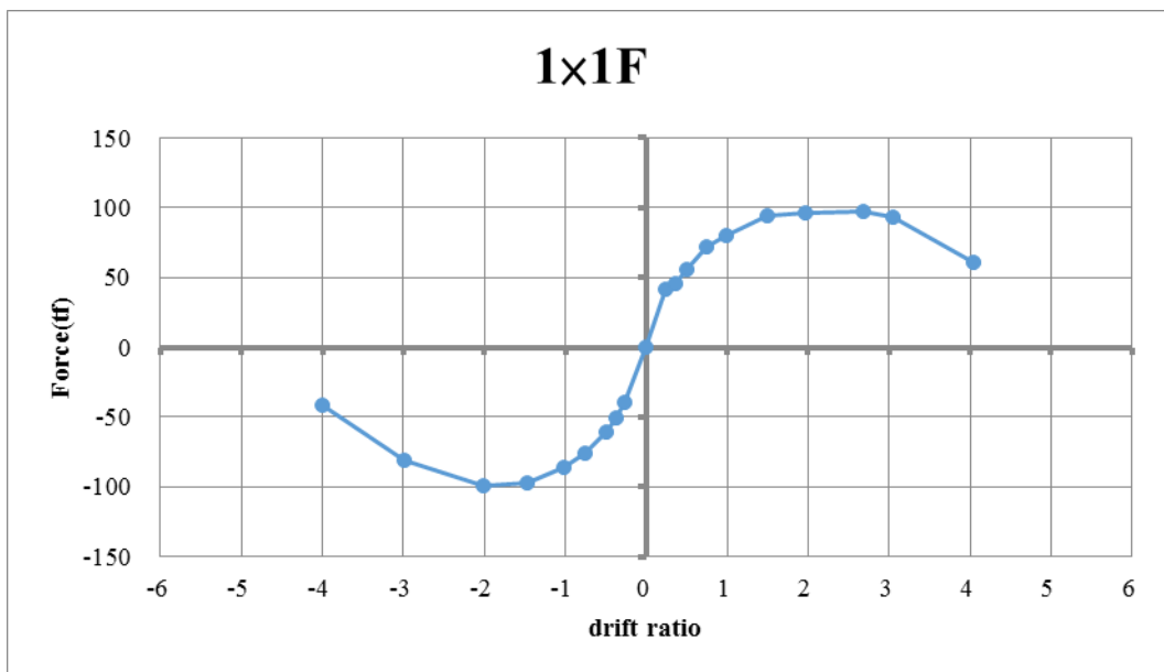
圖 4.6 1x1F 試體遲滯迴圈包絡線
