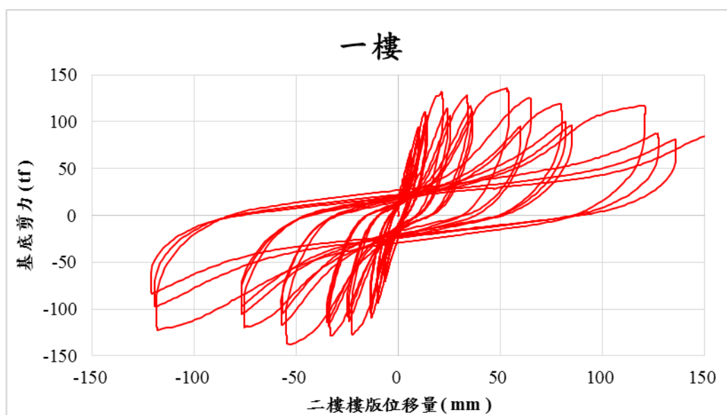
(b) 一樓
