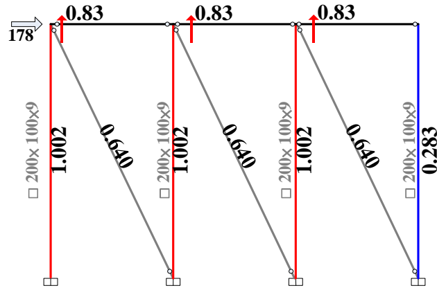
圖 2.6 單層多跨分析之 Strength Ratio(案例二) (資料來源：本研究製作)
