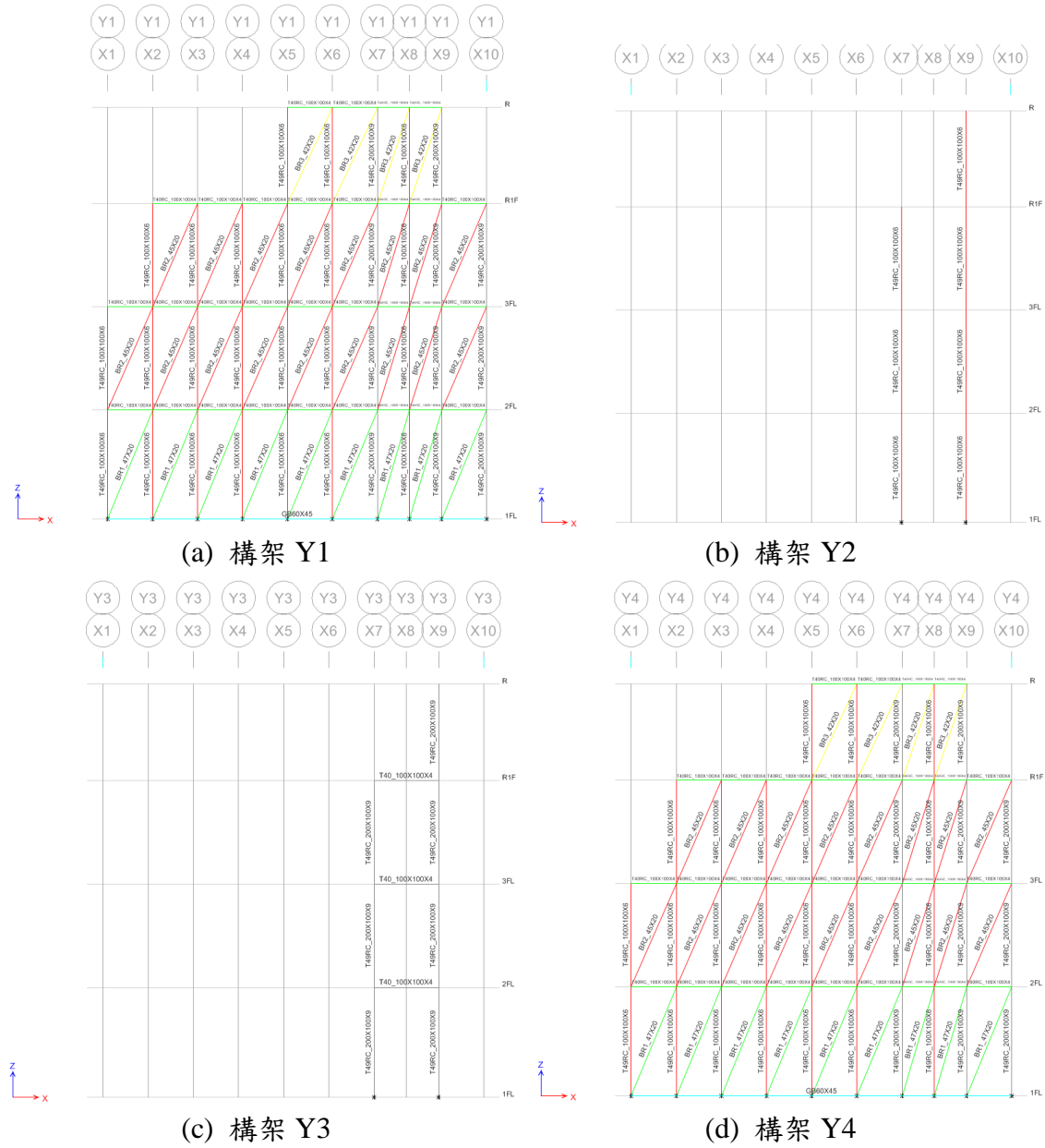
圖 5.9 分析模型構架立面圖
