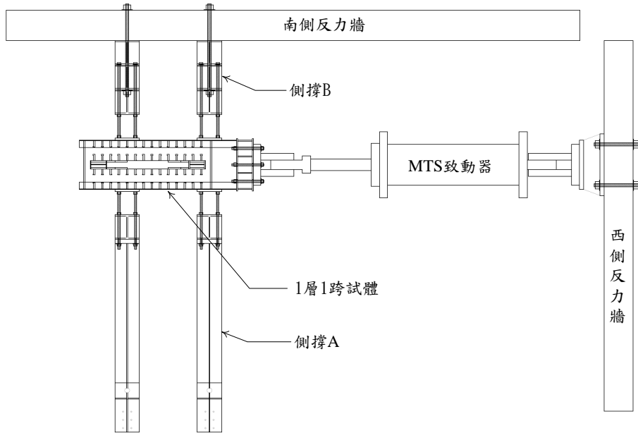
(c) 上視圖
