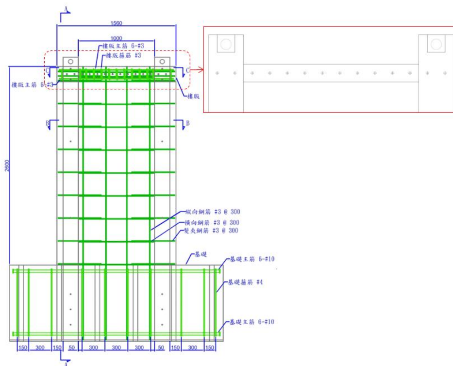
圖 3.2 1x1F 試體示意圖(單位：mm)
