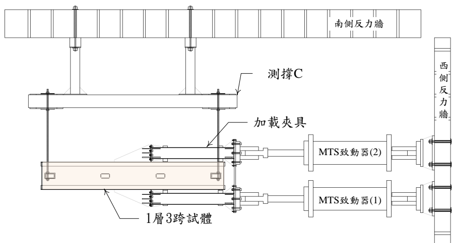
(b) 上視圖
