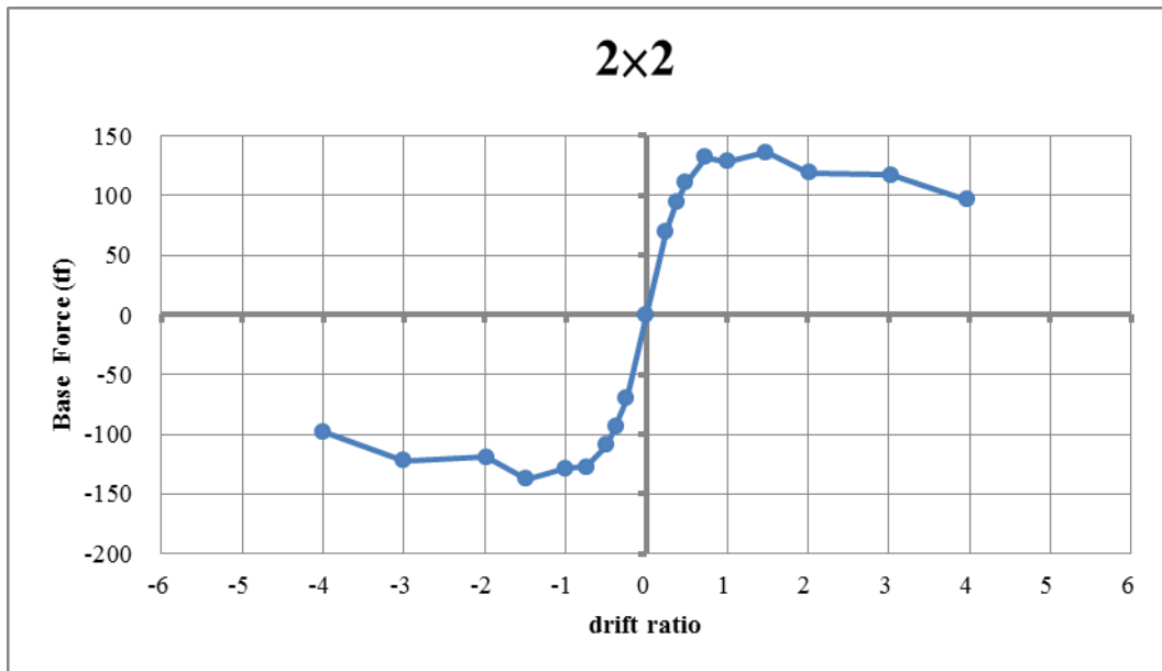
圖 4.20 2x2 試體遲滯迴圈包絡線
