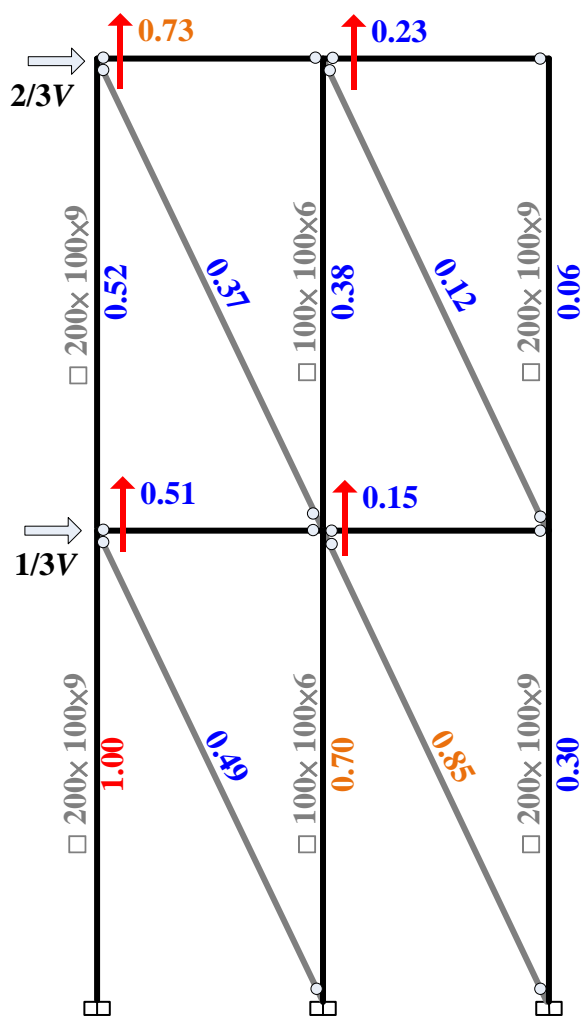
圖 4.27 2x2 構架分析得到之 Strength Ratio
