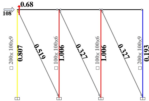
圖 2.5 單層多跨分析之 Strength Ratio(案例一) (資料來源：本研究製作)
