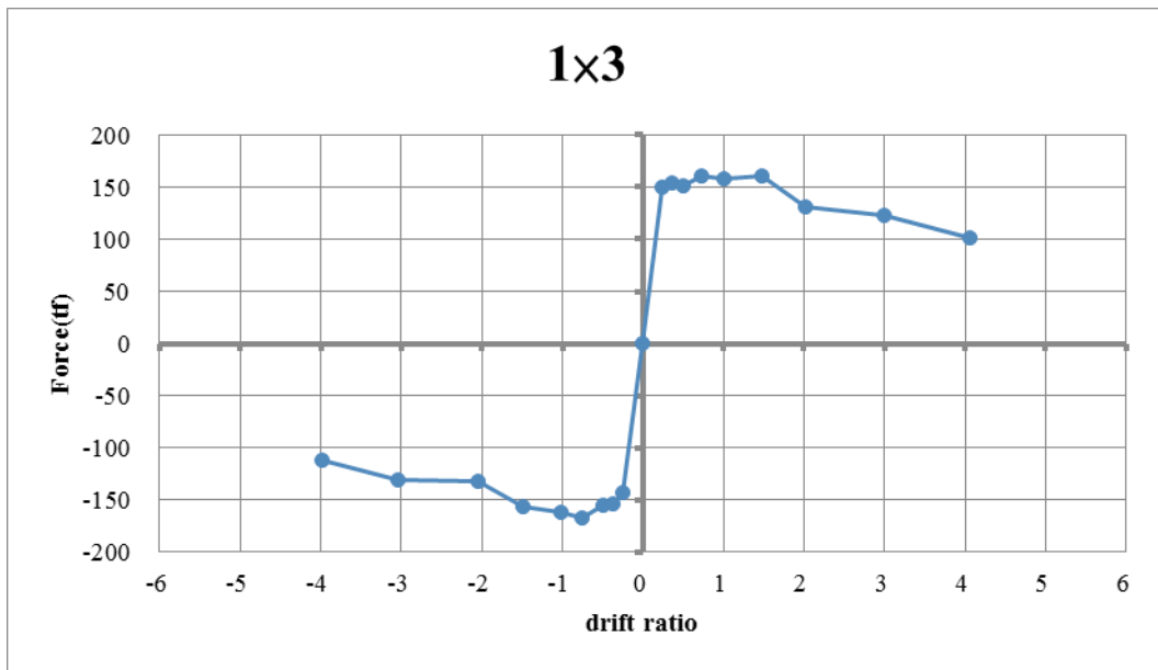
圖 4.14 1x3 試體遲滯迴圈包絡線
