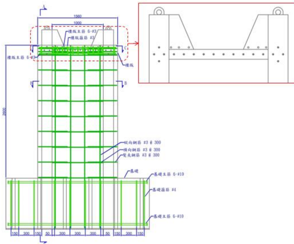
圖 3.1 1x1W 試體示意圖(單位：mm)
