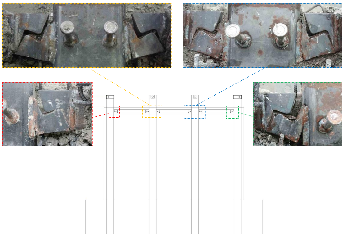
圖 4.18 1×3 試體接頭破壞情況
