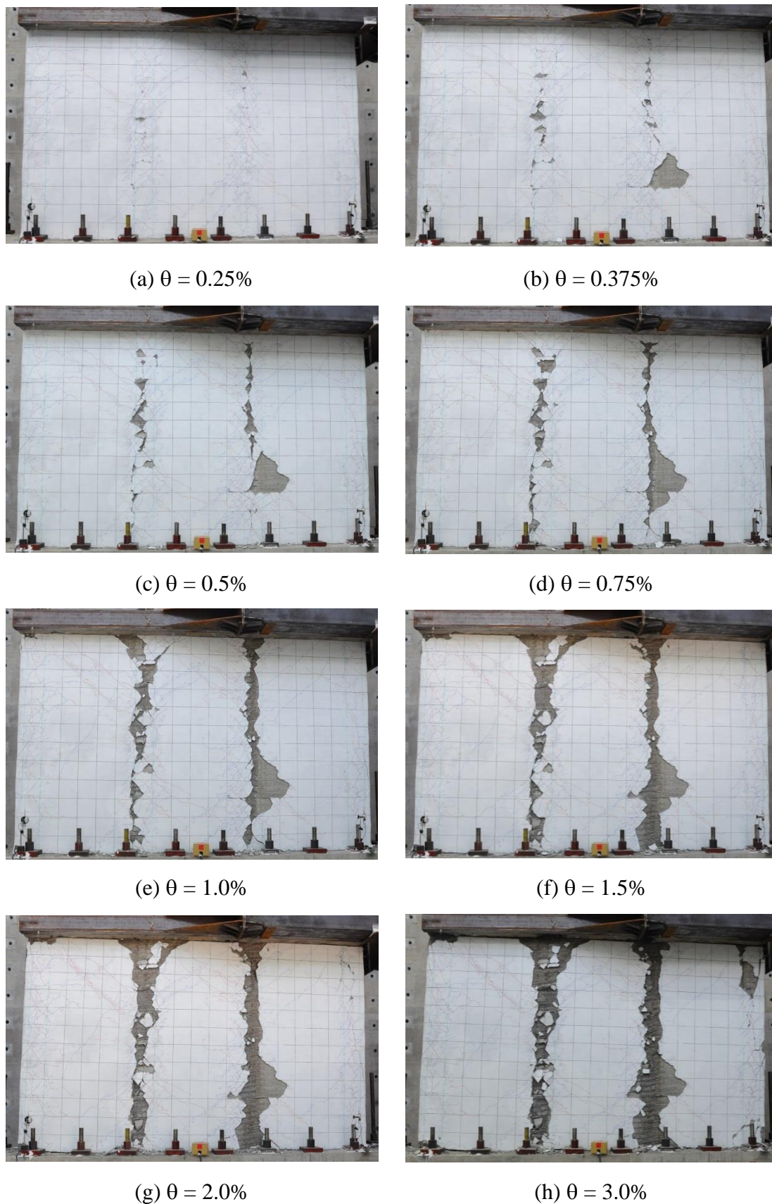
圖 4.15 1×3 試體不同層間位移角試體破壞情況
