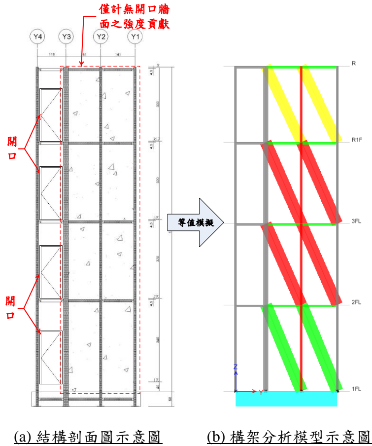
圖 5.2 建築圖、結構圖與分析模型之示意圖
