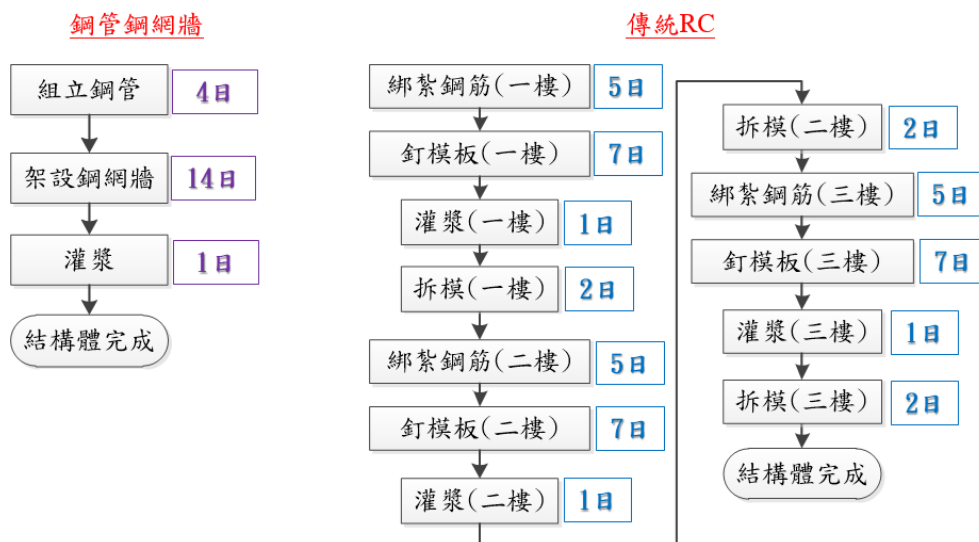
圖 2.1 案例施工流程及時間分析
