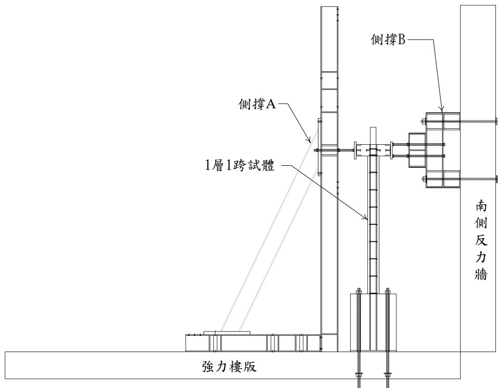
(b) 側視圖
