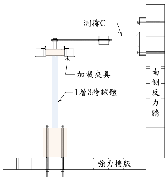
(c) 側視圖
