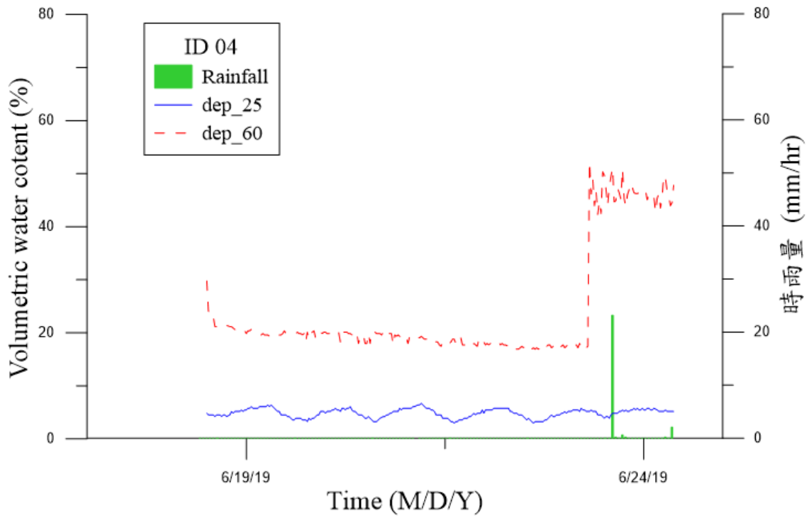
圖 4.13 ID04 體積含水量量測結果
