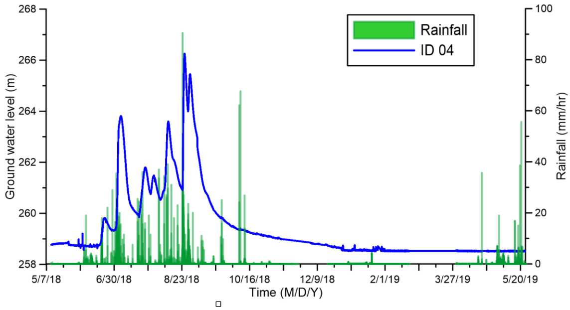
圖 5.6 ID 04 地下水位監測數據
