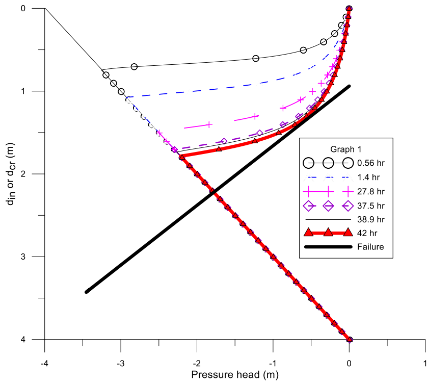
圖 2.14 室內模型試驗壓力水頭與破壞包絡線
