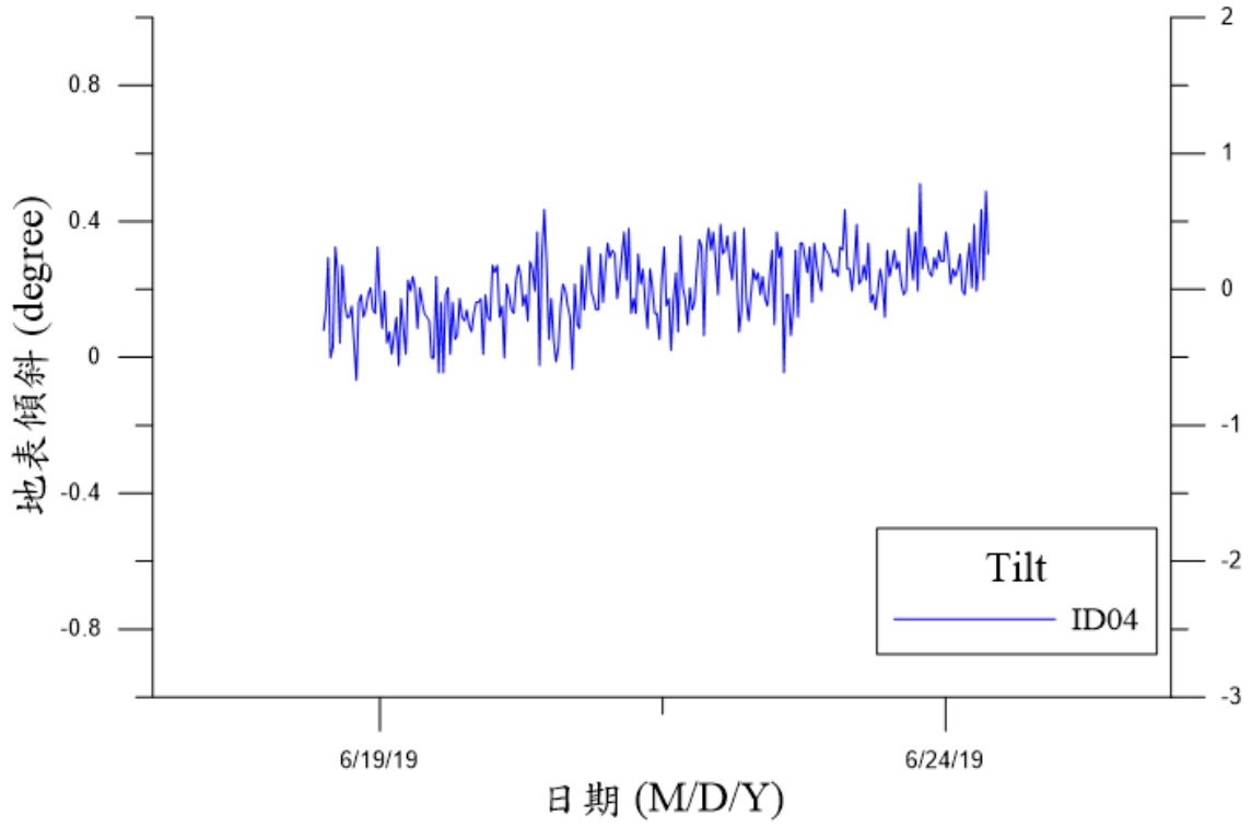
圖 4.16 ID04 傾斜監測結果
