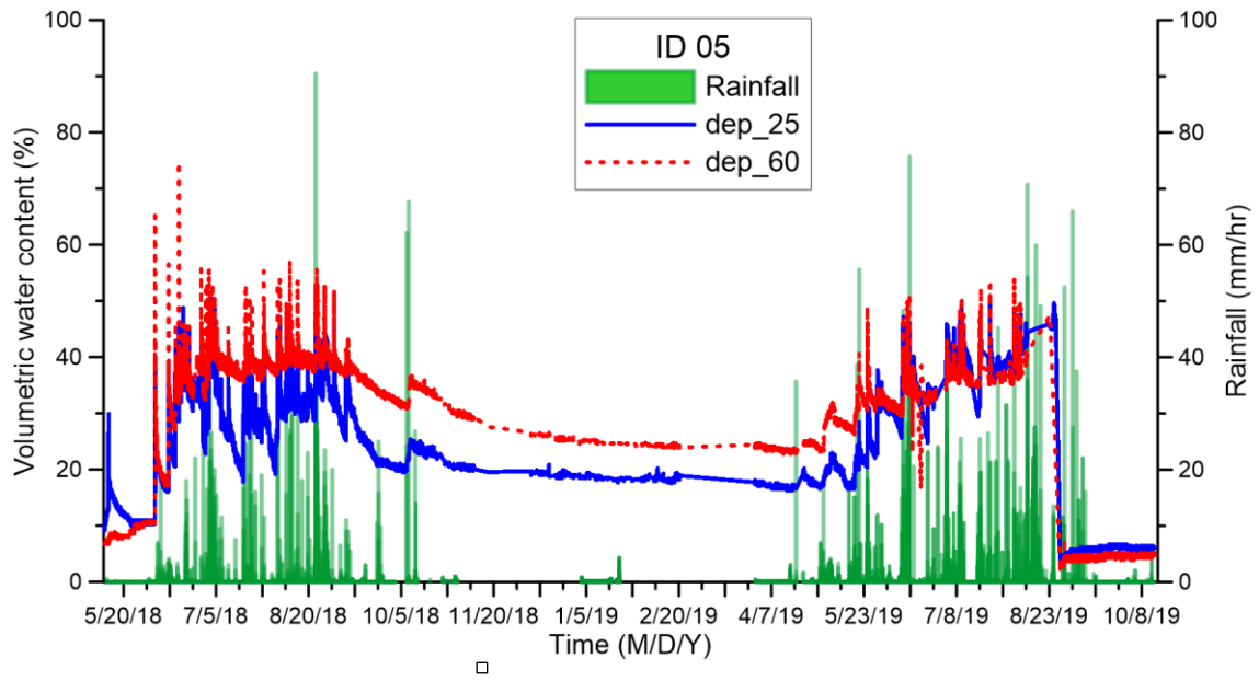
圖 5.15 ID 05 體積含水量監測數據
