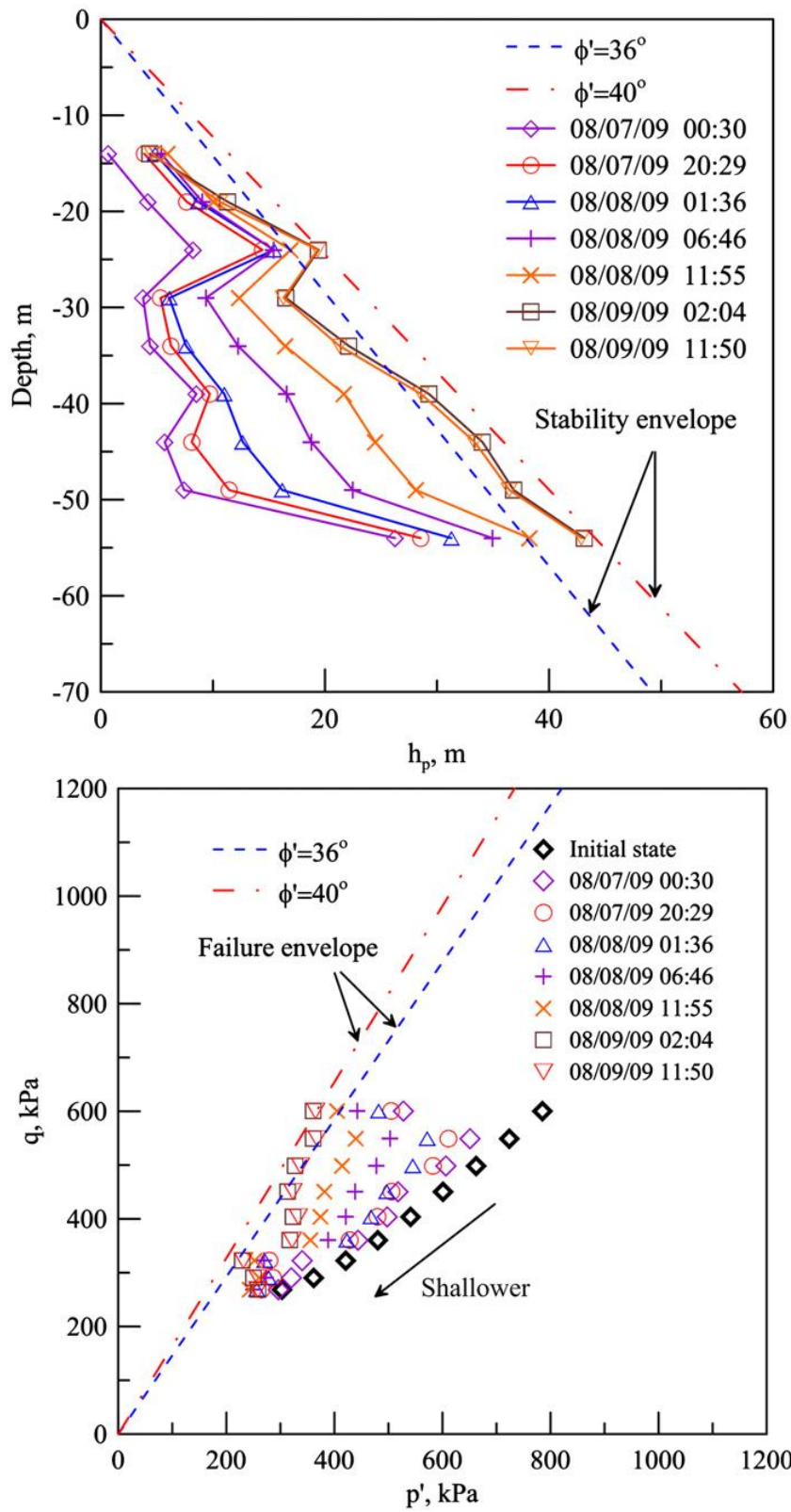
圖 2.2 五彎仔現地孔隙水壓監測與應力路徑圖 (Huang et al., 2012)
