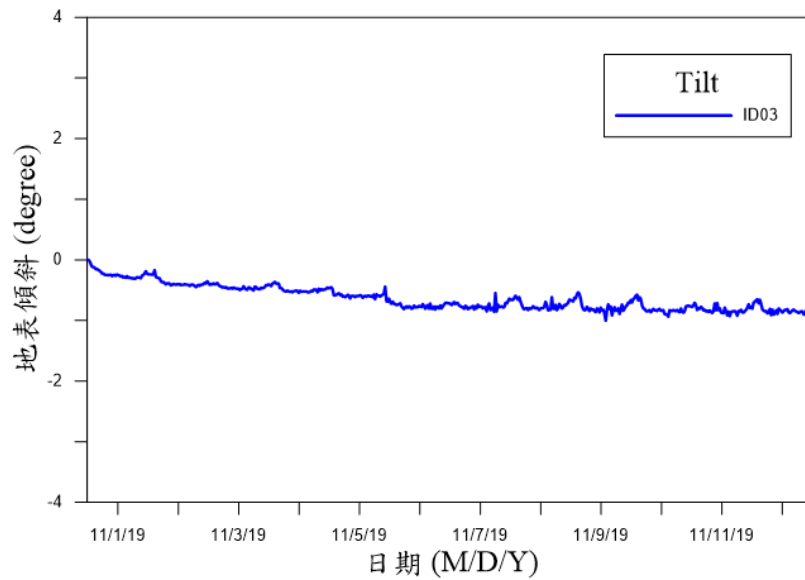
圖 4.24 五彎仔測站修復後 ID3 表面傾斜量測成果
