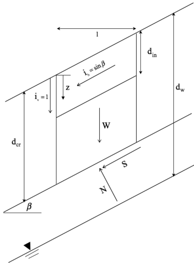
圖 2.7 無限邊坡之水力力學耦合穩定分析示意圖
