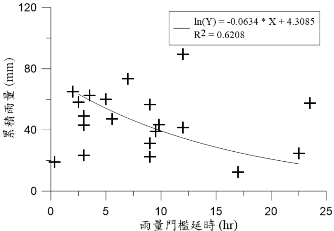
圖 5.11 崩積層雨量門檻延時與累積雨量關係圖
