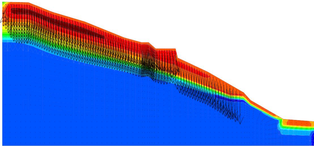
圖 5.18 入滲開始 1.2 \times 10^5 秒孔隙水壓分布與流動向量
