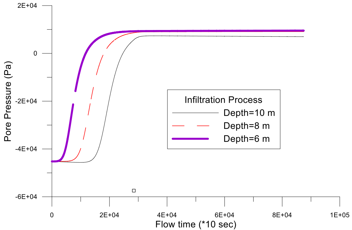
圖 5.21 ID05 位置預測孔隙水壓歷時
