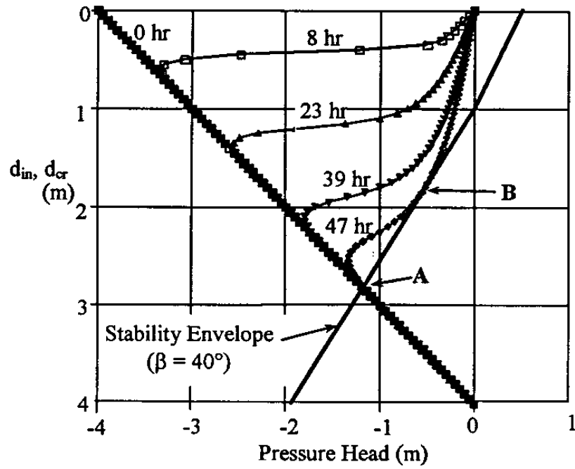
圖 2.3 典型細顆粒土壤入滲分析結果 (Collins and Znidarcic, 2004)
