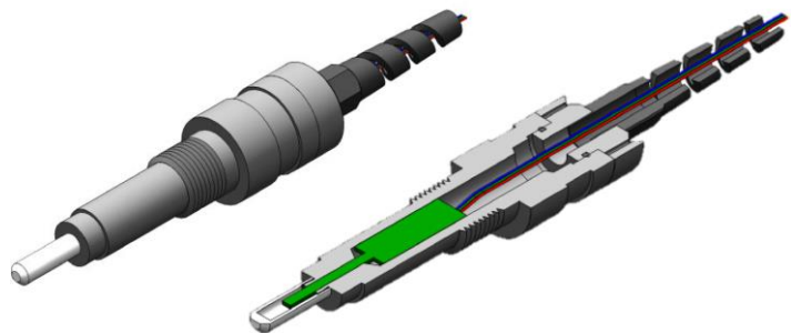
圖 24：溫溼度計防水外殼設計概念圖。
