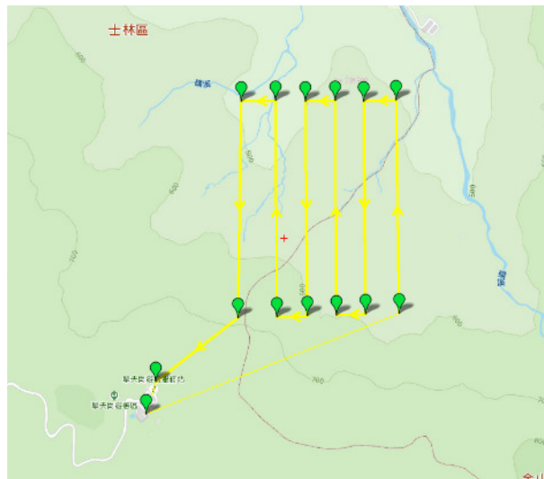
圖 3-2 臺北市士林區(陽明山大油坑)飛行航線規劃
