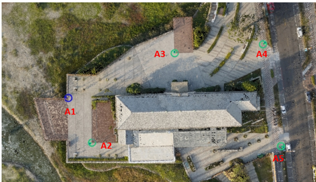
圖 4-34 控制點位置分布
