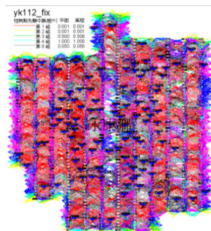
圖 2-30 像片網形連結範例圖
