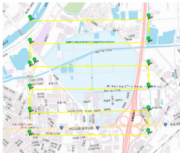
圖 3-13 臺南市永康區飛行航線規劃
