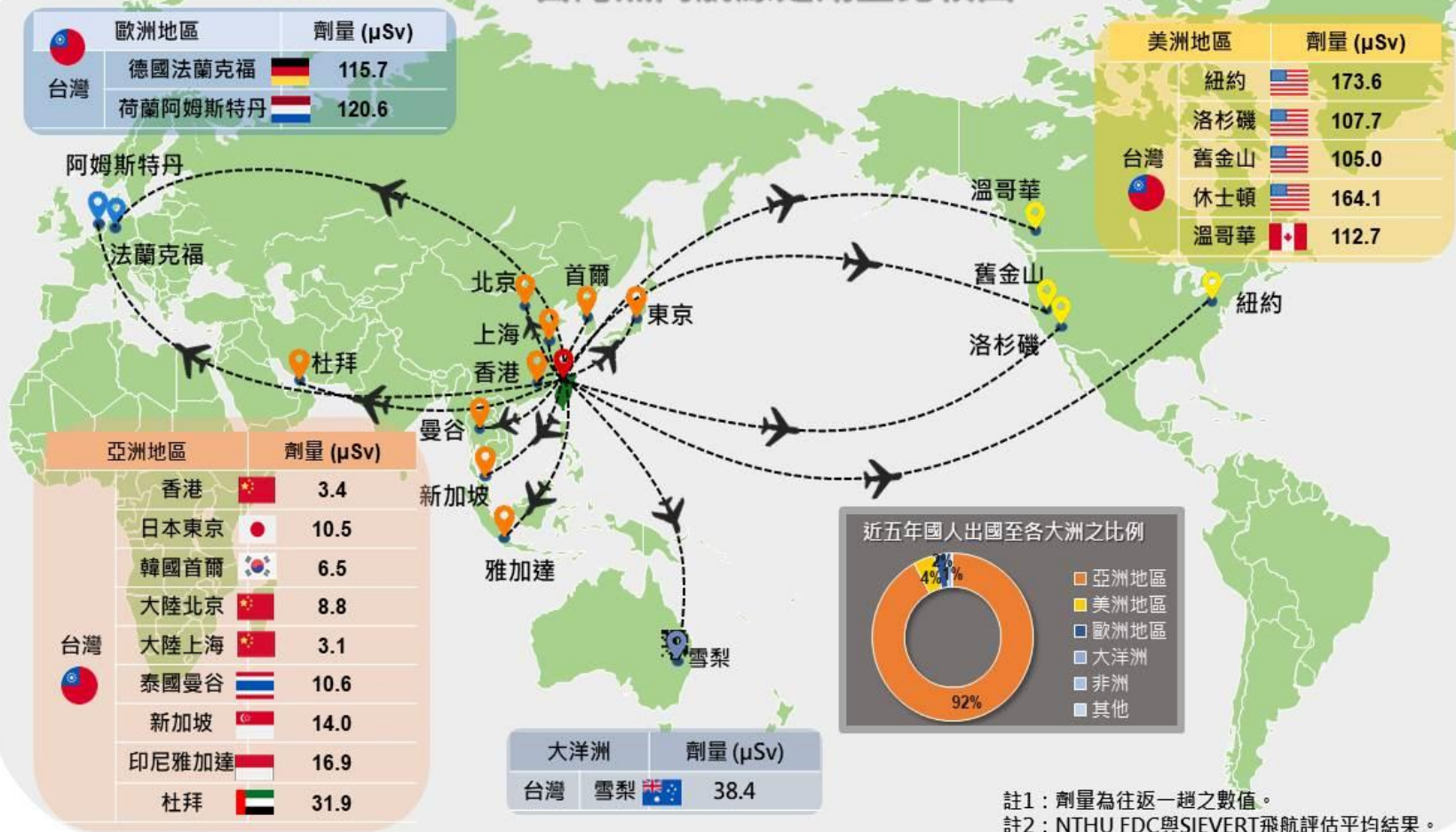
圖 31. 以 NTHU FDC 與 SIEVERT 計算平均值之台灣熱門航線劑量比較圖
