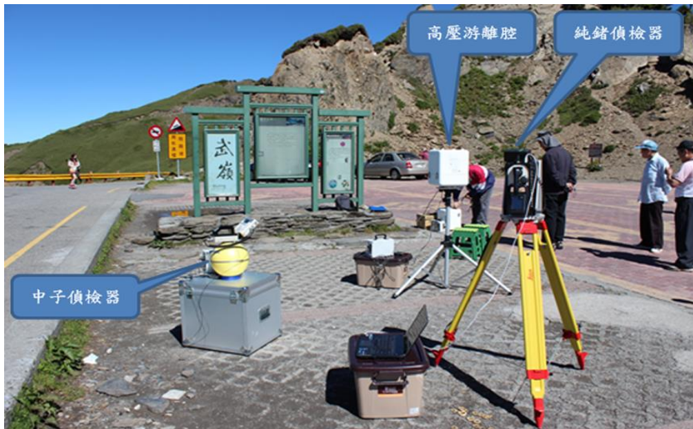
圖 22. 宇宙輻射量測情形(地點：武嶺停車場)
