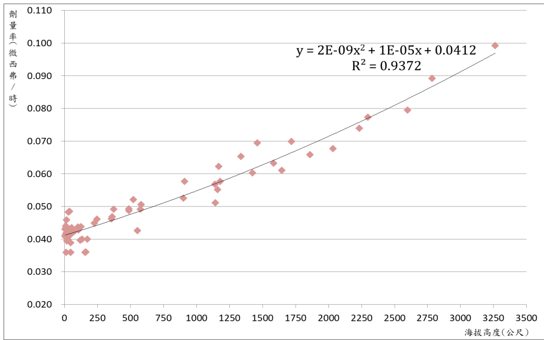
圖 24. 宇宙輻射游離輻射成分劑量率與海拔高度關係
