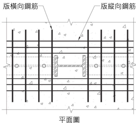
圖 C14.4.2-12 合成部分抗彎矩構架的接合
