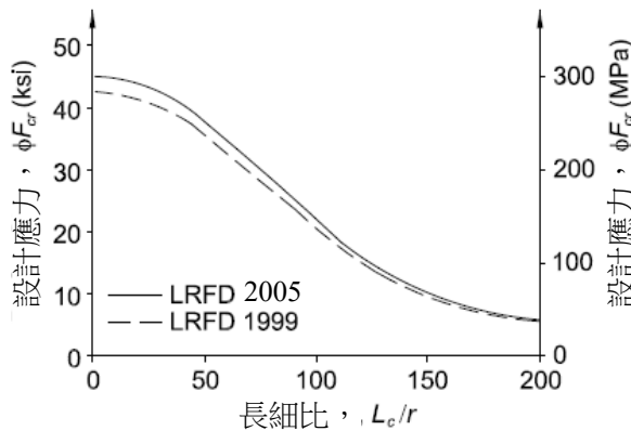
圖 C6.3-1 LRFD 柱曲線比較
