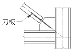
圖C14.11.4-4 挫屈斜撐索引致之載重
