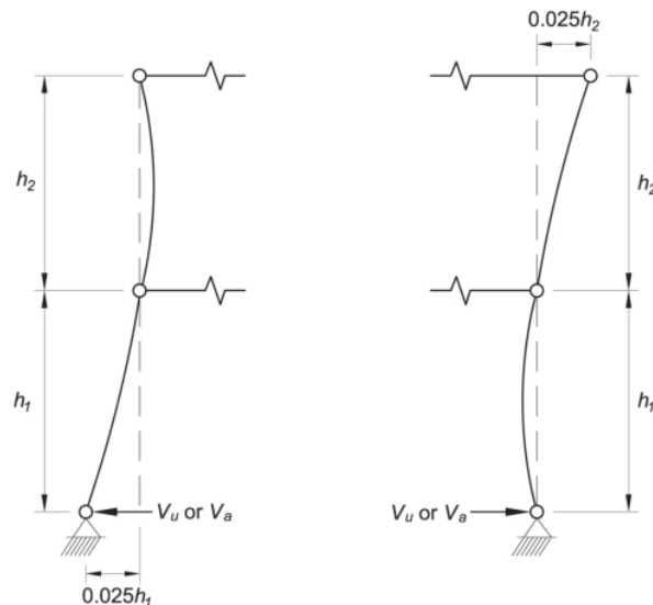
圖 C14.4.2-4 柱位移模型
