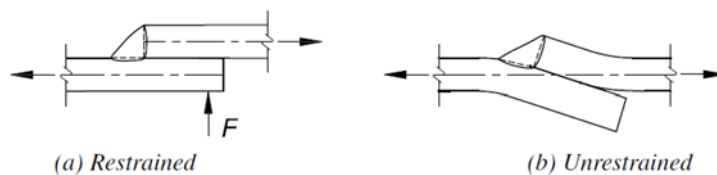
圖C11.2-4 接頭搭限制
