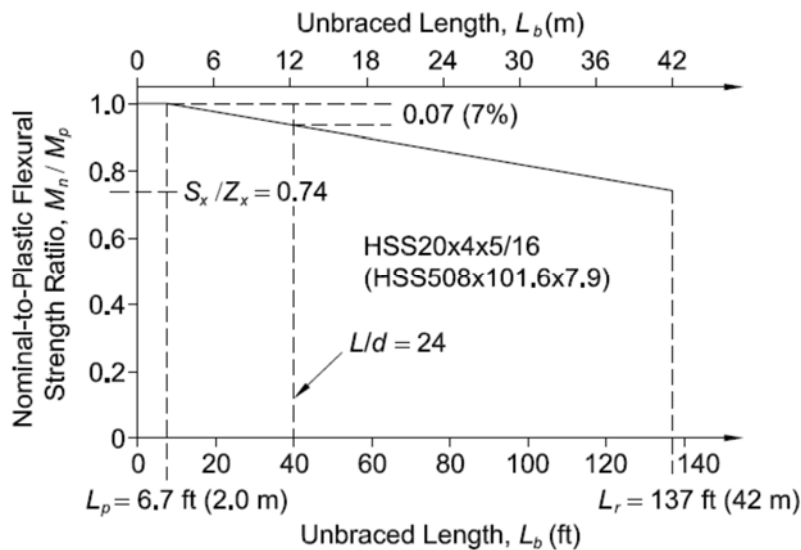
圖 C7.7-1 側向扭轉挫屈之矩形中空斷面 [ F_y = 310 MPa]
