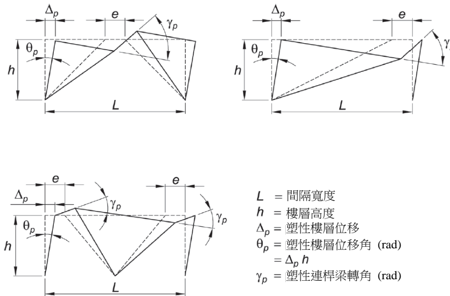
圖C14.12.4-1 連桿轉角
